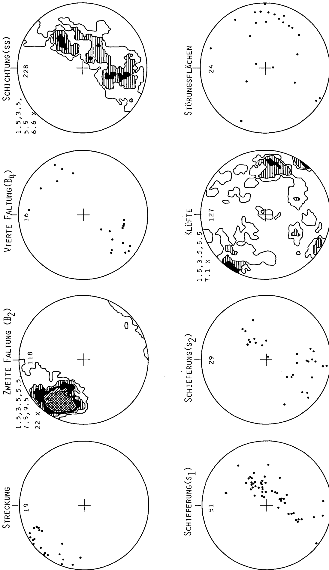
Abb. 2: Orientierungsdaten aus der Veitscher Decke im Bergbaurevier. Schmid'sches Netz, Computerkonturierung nach BEASLEY (1981): gemessenes Gefügeelement über N-Punkt, Zahl rechts oben Diagrammnummer, Konturierungsintervalle (pro 1%) links oben, darunter Bezeichnungsdichte des Maximums (+). Die s 2 und s 1 -Flächen spiegeln die D 2 -Faltung wieder. Die s 2 -Flächen stehen gewöhnlich steil auf (bzw. s 1 ). Unter der Annahme, daß die Flächen Ebenen senkrecht zur D 2 -maximalen Verkürzungsrichtung markieren, ist die D 2 -Einengungsrichtung gegeben. Weitere Erläuterungen im Text.
