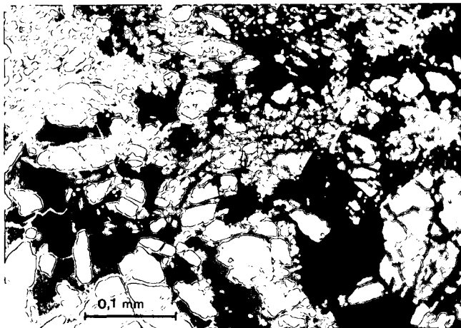
Abb. 6: Die gemeinsame Deformation von Gesteins- und Erzparagenese führte im weniger plastischen Arsenkies (weiß) zu einer intensiven Kataklase. Ausgehend von den Fragmentengrenzen ist der Arsenkies durch Einflüsse der Oxidation umgewandelt zu Limonit (grau). Polierter Anschliff vom Rauhen Kopf, 1 Nicol.
