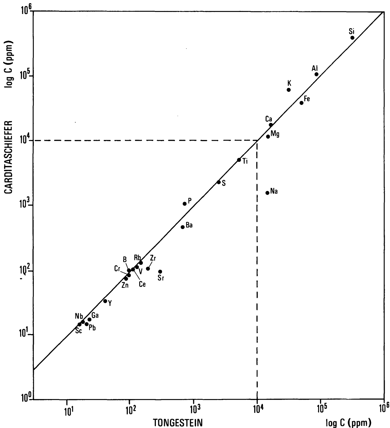
Abb. 1: Vergleich Carditaschiefer/Tongestein nach TUREKIAN & WEDEPOHL (1961).
