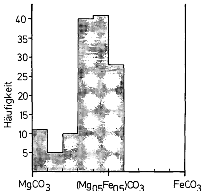
Abb. 1: Histogramm. Die Häufigkeit ist gegen die Zusammensetzung der Magnesit-Siderit-Mischkristalle aufgetragen. 135 Punktanalysen, die an jeweils 2 Anschliffen von 5 verschiedenen Karbonatgesteinsproben durchgeführt wurden.
