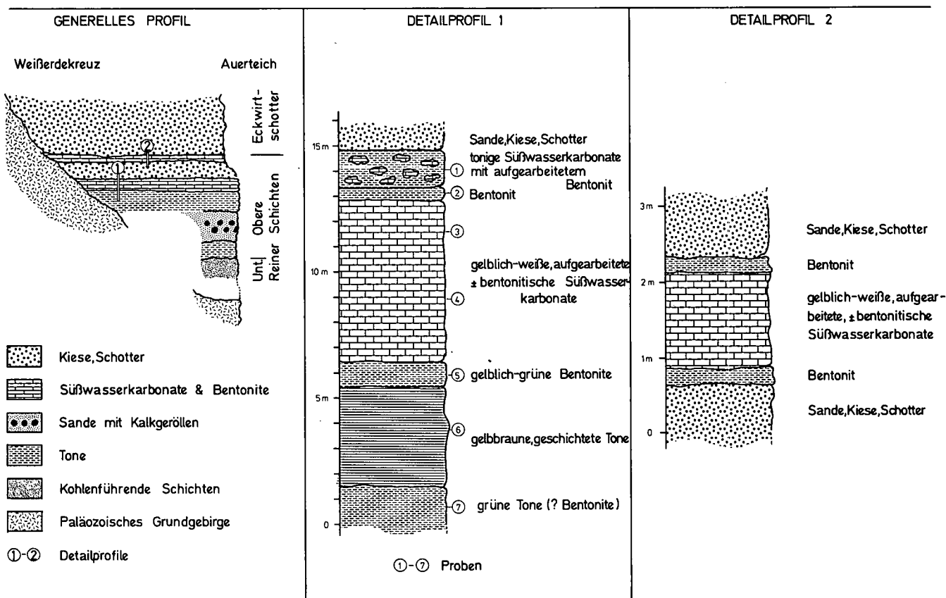
Abb. 18: Fazielle Entwicklung im Reiner Becken (F. EBNER &amp; W. GRÄF, 1982).
