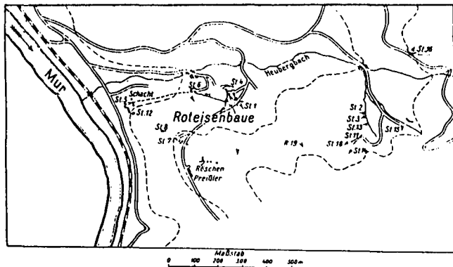
Abb. 4: Lage der Baue auf Hämatit und Manganerze im Heuberggraben bei Mixnitz (nach E. SEIDLER aus K. A. REDLICH, 1931).
