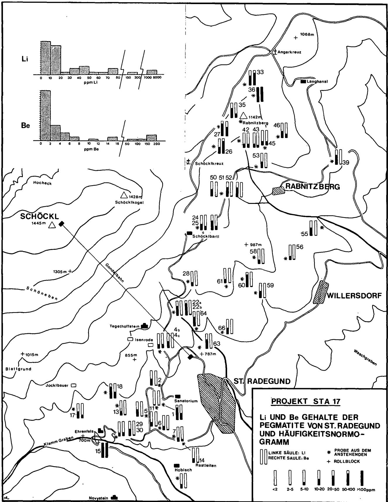
Abb. 1: Lithium- und Beryllium-Gehalte der Pegmatitproben von St. Radegund (F. KOLLER et al., 1983). Maßstab: Strecke der Gondolbahn = 2 km.
