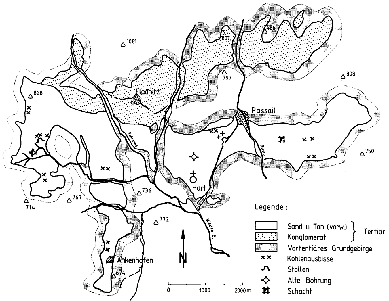
Abb. 13: Geologische Übersichtskarte des Passailer Tertiärbeckens (L. WEBER &amp; A. WEISS, 1983).
