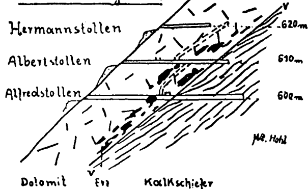
Abb. 5: Schematisches Profil durch den Fahlerzbergbau im Wetterbauergraben bei Mixnitz (O. HOHL, 1929).
