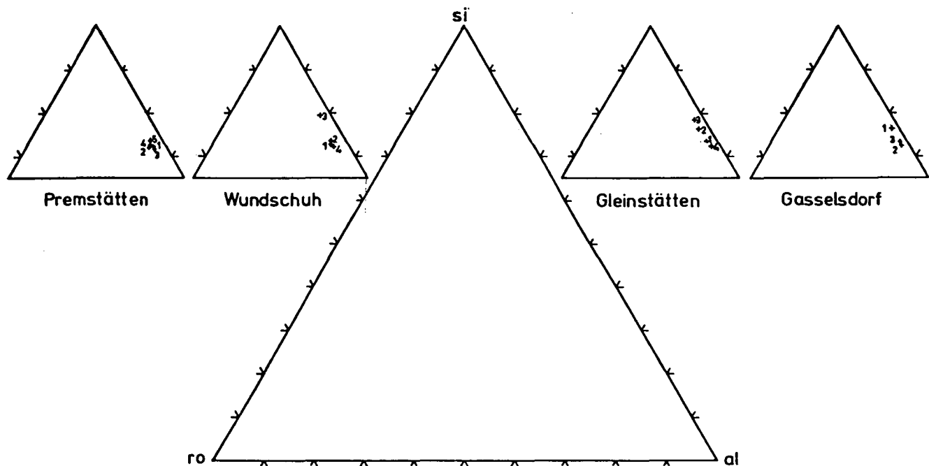
Abb. 25: Diagramm si – ro – al für Rohstoffe der Ziegeleien Premstätten, Wundschuh, Gleinstätten und Gasselsdorf (J. G. HADITSCH & F. LASKOVIC, 1974; modifiziert).
