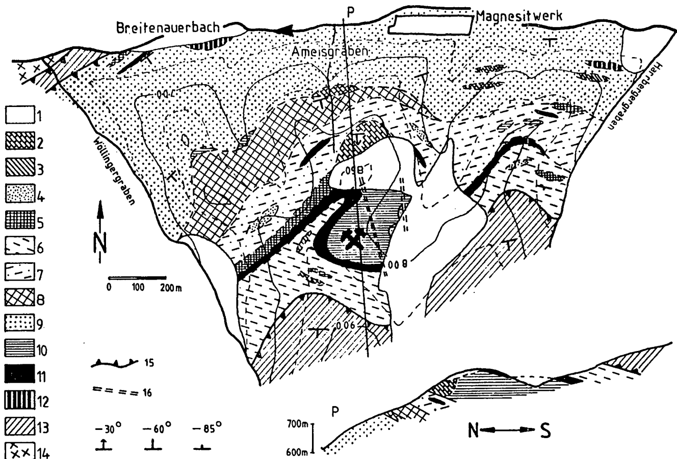
Abb. 20: Geologische Karte und Profil (P) am Hochlantsch, Nordabfall im Bereich der Magnesitlagerstätte Breitenau (H. GOLLNER et al., 1982). 1 = Hangschutt, Halde; 2 = Kalk; 3 = Dolomit; 4 = Sandstein; 5 = Lydit; 6 = Tonstein (oberer Anteil der Hackensteiner-Formation); 7 = Tonstein (mittlerer Anteil); 8 = Lydit/Tonstein-Wechselfolge; 11 = Metatuffit; 12 = Metabazit; 13 = Kalkschiefer-Folge; 14 = Kristallin; 15 = Überschiebung; 16 = Störung.
