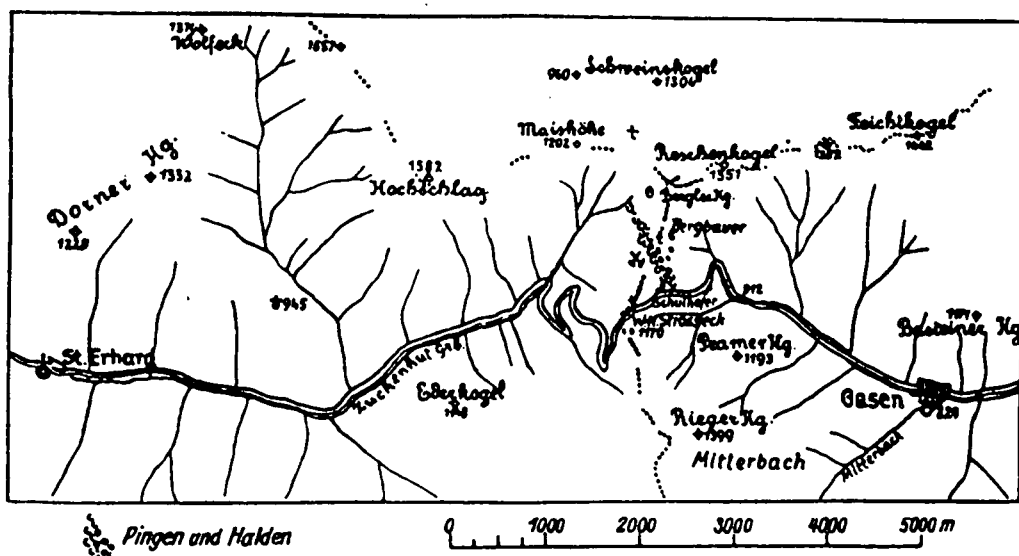
Abb. 7: Lageskizze des Bergbaues auf dem Straßbeck-Sattel (F. CZERMAK &amp; J. SCHADLER, 1933).
