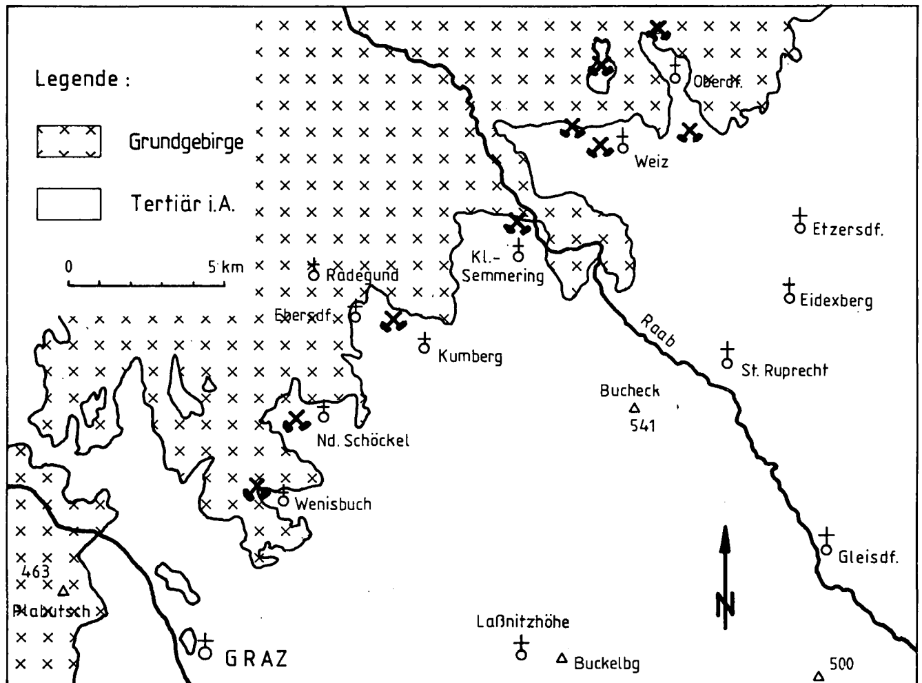
Abb. 12: Lage der Braunkohlenvorkommen der Grazer Bucht (L. WEBER &amp; A. WEISS, 1983).
