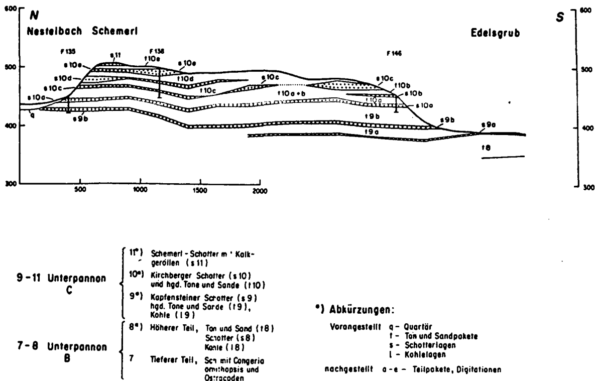
Abb. 24: Schotterlagen des Unterpannon des Steirischen Beckens (K. KOLLMANN, 1964; modifiziert).
