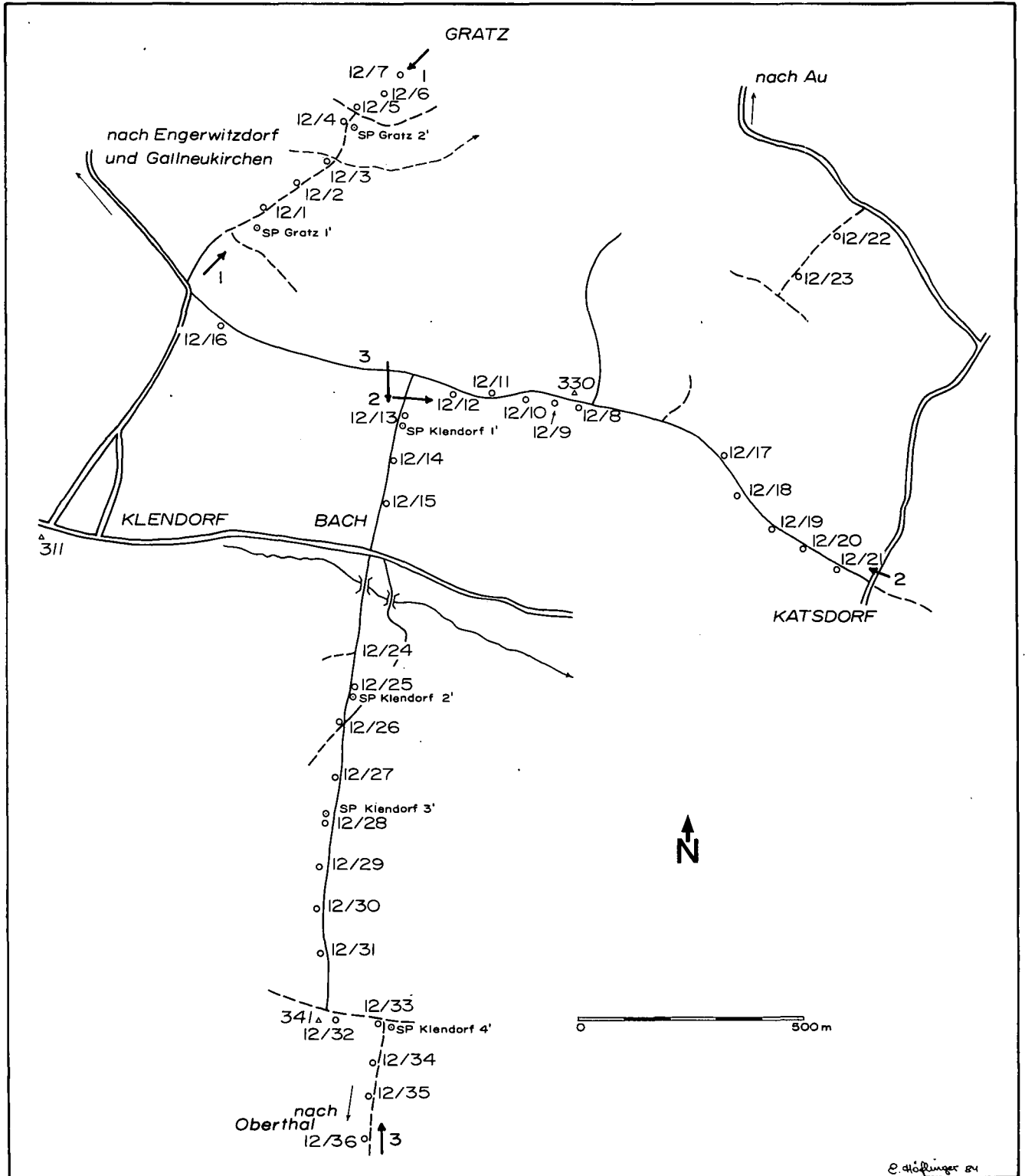
Abb. 21: Lageplan der geoelektrischen Tiefensondierungen, refraktionsseismischen Profile und der geologisch-geophysikalischen Profilschnitte im Raum von Gratz und Katsdorf.
