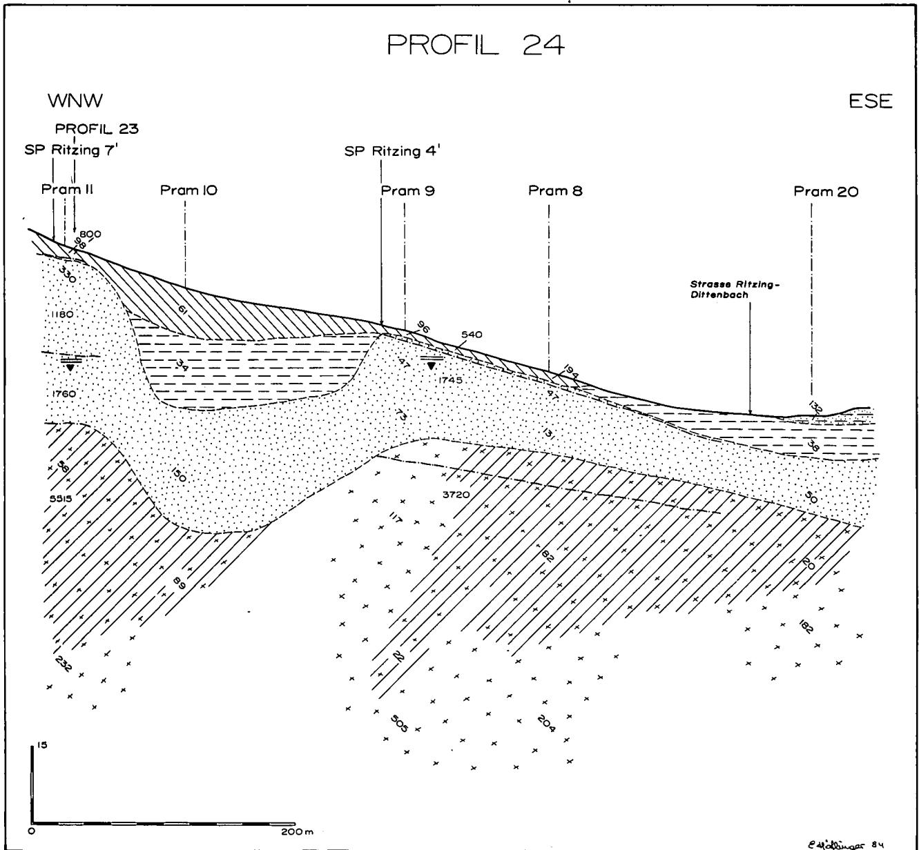
Abb. 7: Geologisch-geophysikalischer Profilschnitt 24 aus dem Bereich Ritzing/Manzing. Legende siehe Abb. 3; Lageplan siehe Abb. 5.
