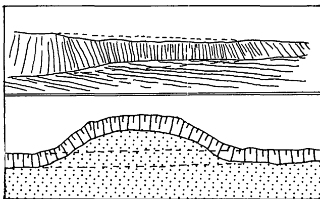
Abb. 3: An die Topographie angepaßte Abbauform mit konkaver, verschliffener Abbaufront.
