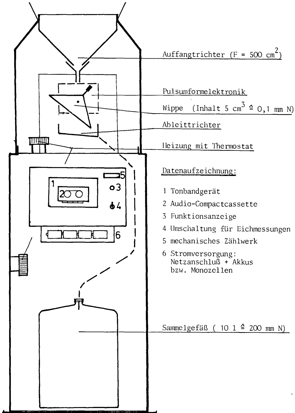
Abb. 1: Automatisches Niederschlagsmeßgerät.
