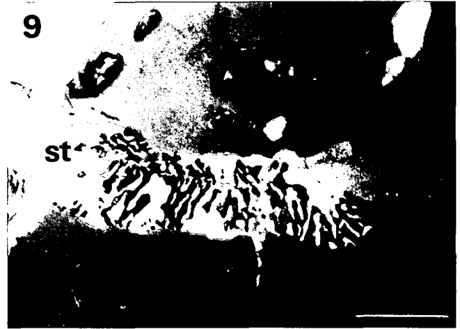
Abb. 13. Myrmekitbildung bei Antimonit – ged. Antimon (im Bild nicht erkennbare winzige Tröpfchen) – Pyrrhotin, daneben Tetraedrit. Abkürzungen siehe Abb. 4. Nicols +.
