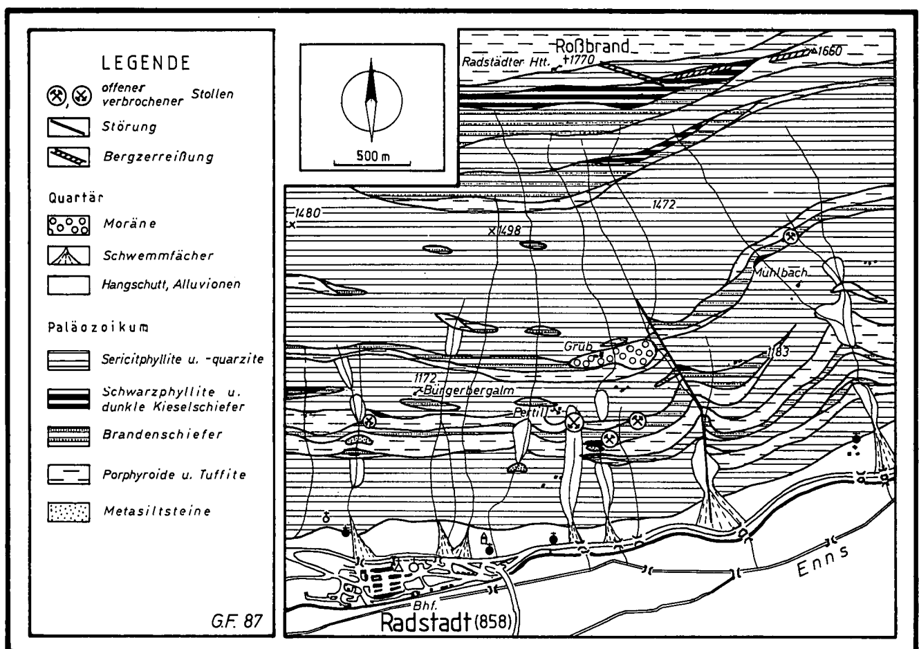
Abb. 3. Geologische Karte der Grauwackenzone im Bereich Radstadt - Schwemmberg.
