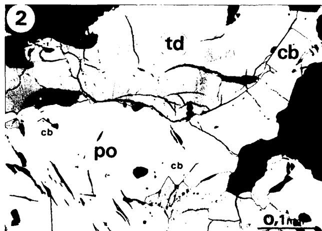
Abb. 6. Idiomorphe Cobaltin-Kristalle ({100} vorherrschend) in Pyrrhotin und Tetraedrit. Abkürzungen siehe Abb. 4.
