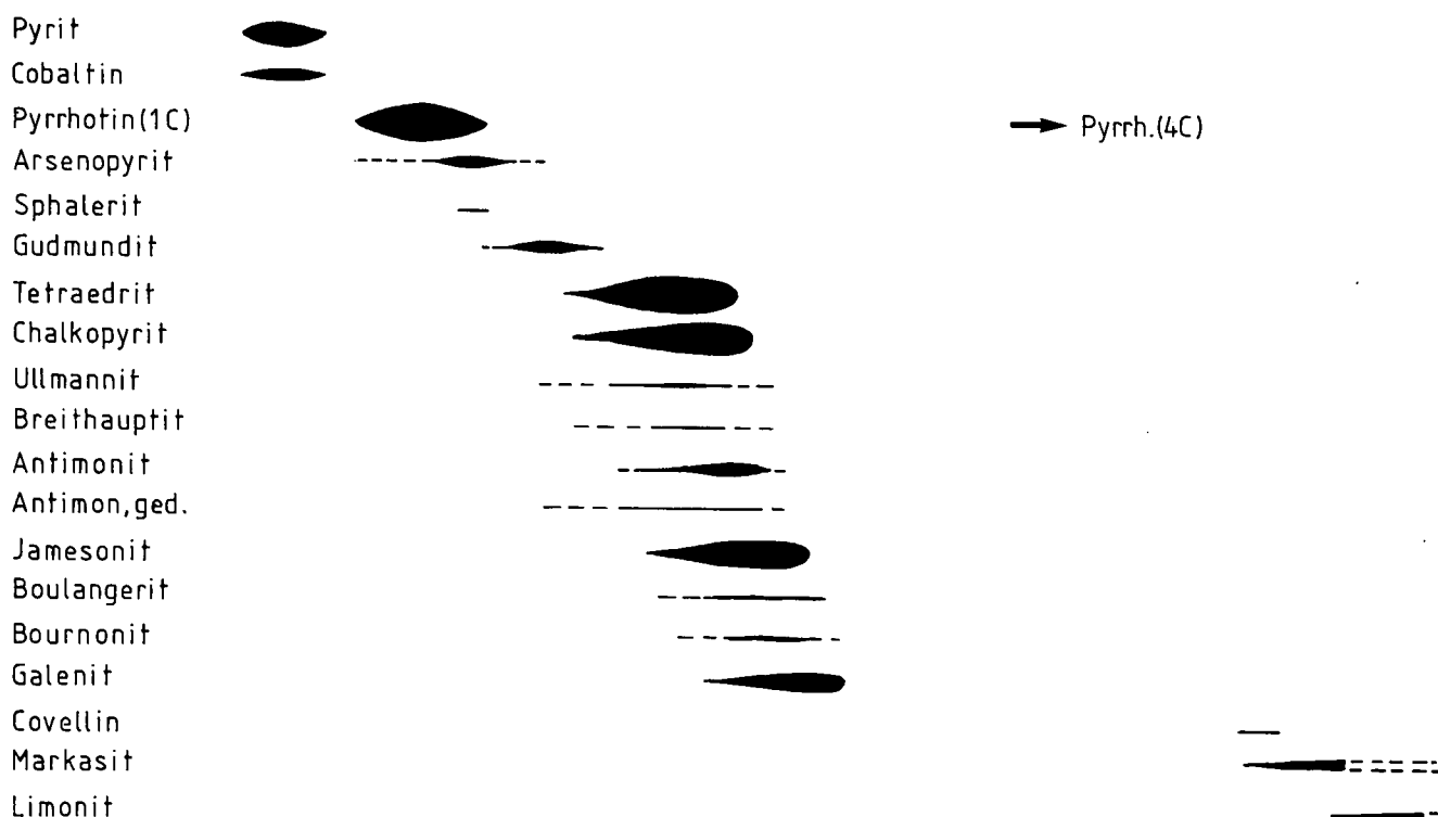
Abb. 16. Kristallisationsschema der komplexen Cu(Ag,Hg)-Fe-Co(Ni)-Pb(Zn)-As-Sb-Sulfidparagenese. Die Dicke der Linsen soll die relative Häufigkeit des jeweiligen Minerals andeuten.
