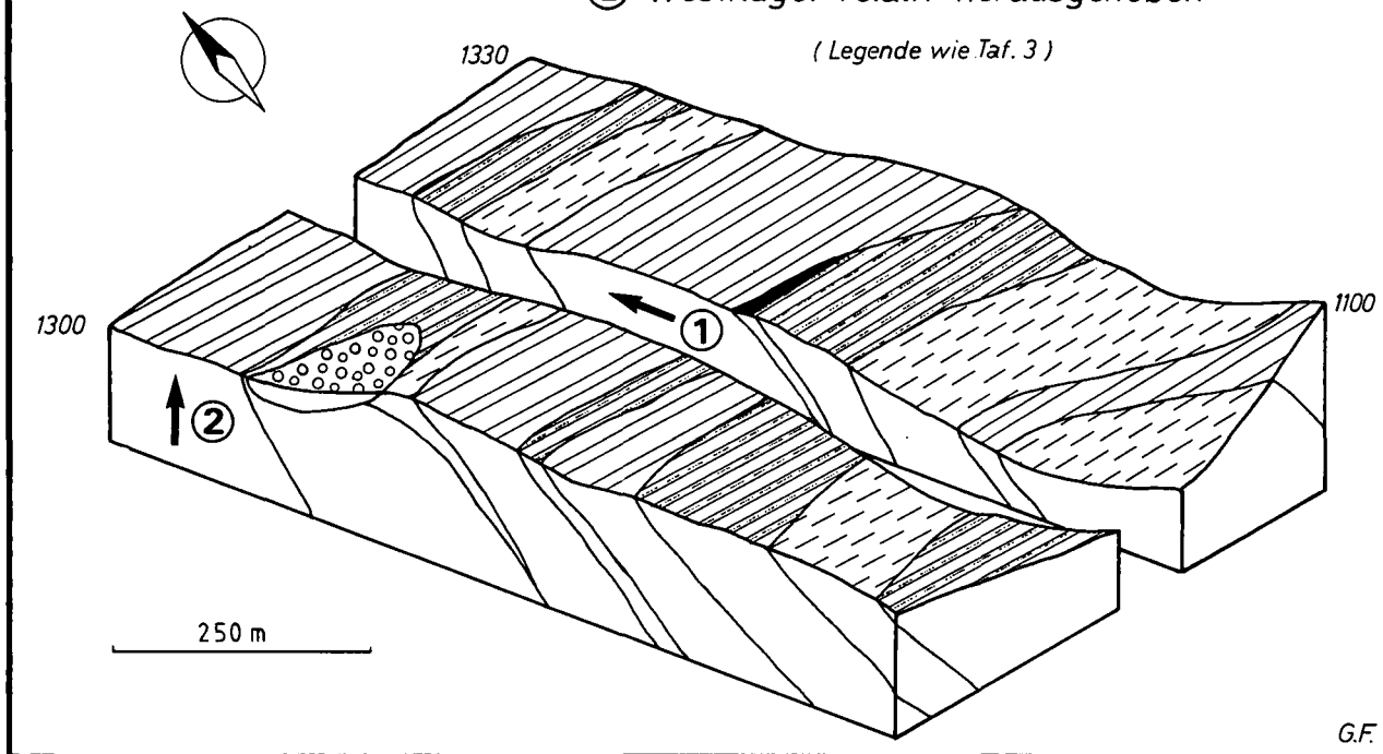
Abb. 5. Möglichkeiten tektonischer Verstellungen im Mittelteil des Höllgrabens.
