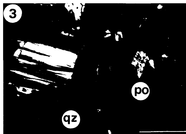
Abb. 7. Deformation bei Pyrrhotin. Erkennbar sind Knickbänderung und Zwillingslamellierung. Abkürzungen siehe Abb. 4. Nicols +.
