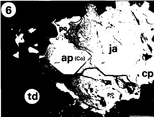
Abb. 10. Jamesonit verdrängt Pyrrhotin; daneben Chalkopyrit und Tetraedrit. Jamesonit umwächst einen hypidiomorphen Kristall von Co-hältigem Arsenopyrit (Danait). Abkürzungen siehe Abb. 4.
