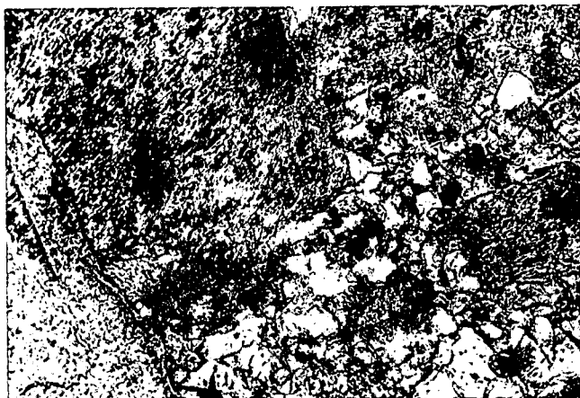
Abb. 6. Kaolinsand. Lokalität: Bohrloch 3, Tiefe 19,8 m; Probennummer BL-3/28; Bildausschnitt 3,36 x 2,21 mm; Nicols ||. Grauweiß = Quarzkörner in kaolinitischer Matrix (hellgrau bis grau).
