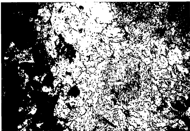
Abb. 5. Kaolinisierter Granulit aus autochthoner Zersetzungszone. Lokalität: Bohrloch 3, Tiefe 20,5 m; Probennummer BL-3/26; Bildausschnitt 3,36 x 2,21 mm; Nicols ||. Grauweiß = Quarz; grau bis dunkelgrau = fast vollständig kaolinisierte Feldspäte; Granulitgefüge noch deutlich zu erkennen.
