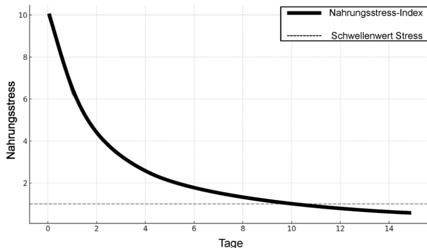
Abb. 4: Entwicklung des Nahrungsstress ( \text{FoodStress}(t) = D_{\text{tot}}(t)/F_{\text{tot}}(t) ) mit der Zeit. Der Schwellenwert markiert niedrigen Stress infolge eines Überangebots an Nahrung in Bezug auf die Populationsgröße.
