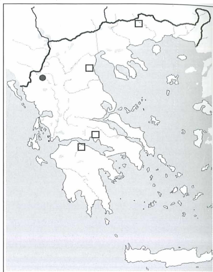
224. Apamea illyria (FRR.)
