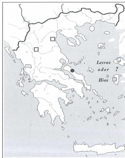
113. Cucullia lychnitis (RAMBUR)
