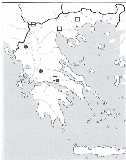
225. Apamea anceps (D. & S.)
