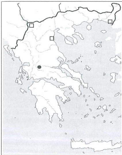
245. Lacanobia suasa (D. & S.)
