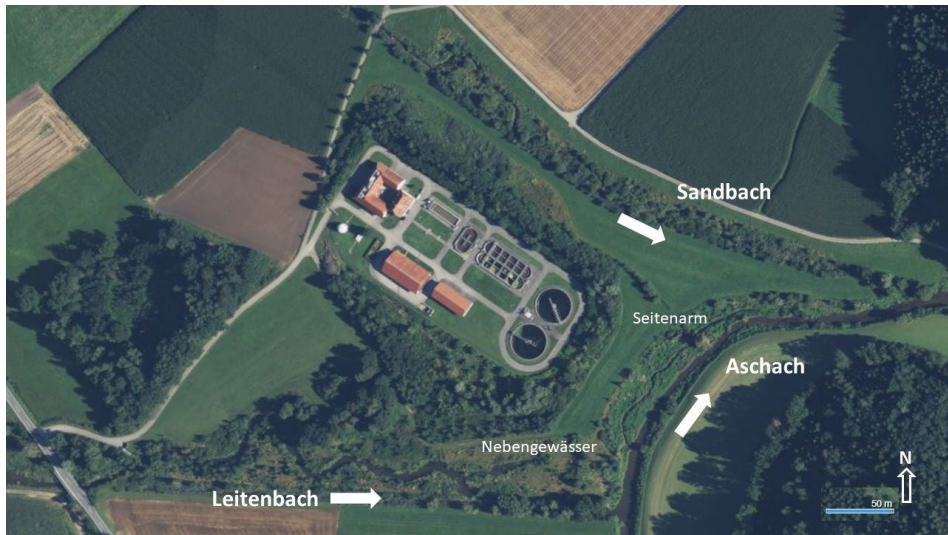
Abb. 1: Das Untersuchungsgebiet: Unterläufe und Mündungen von Leitenbach und Sandbach in die Aschach nach Durchführung der Restrukturierungsmaßnahmen. / The investigation area: lower sections and mouths of Leitenbach and Sandbach into the Aschach after the implementation of the rehabilitation measures. Quelle: https://www.bing.com/maps .
