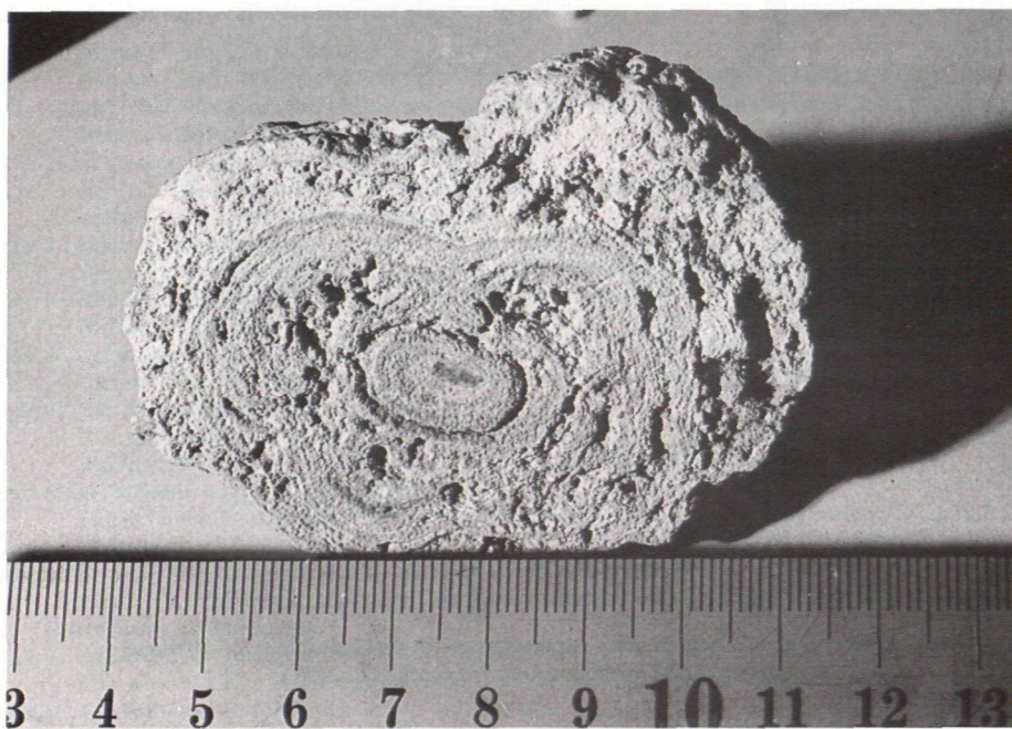
Abb. 3: Kleiner Onkoid im Längsschnitt.
