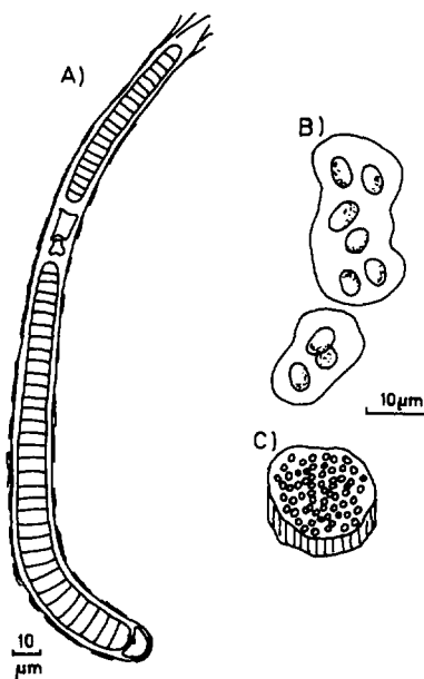
Abb. 6: Weitere Blaualgen aus den Kalkbildungen, A) Calothrix gypsophila , B) Aphanothece saxicola , C) Microcystis anodonta .
