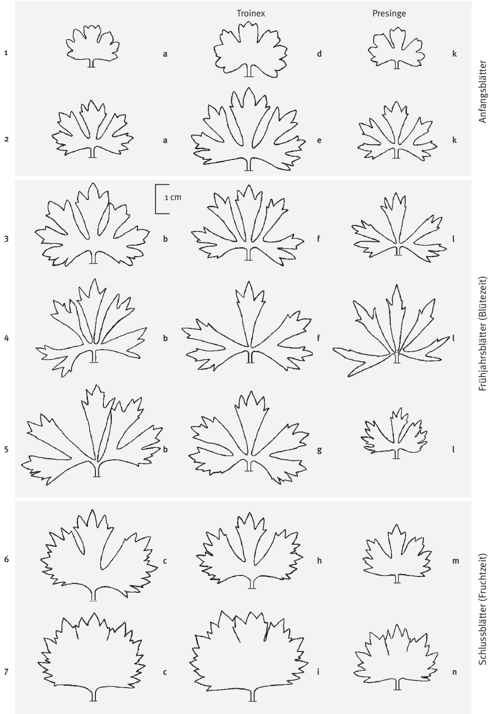
Abb. 6: Grundblattzyklus von Ranunculus moorii .
