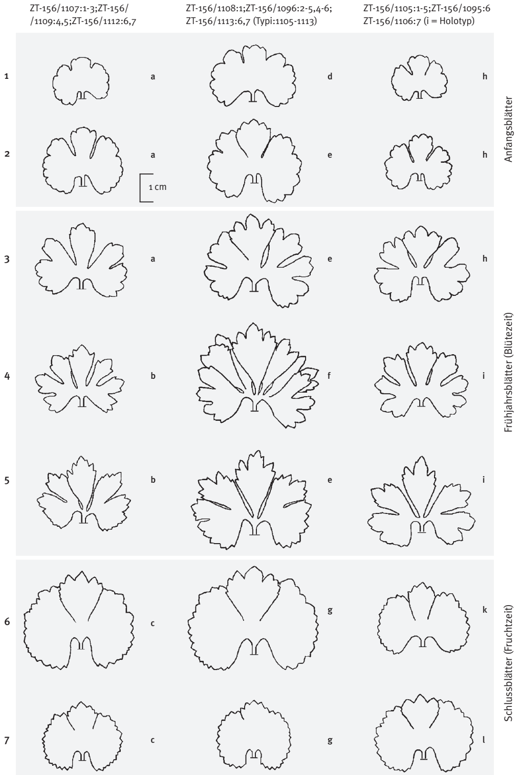
Abb. 5: Grundblattzyklus von Ranunculus hirsutulus . 1–7: Grundblattfolge im Jahresverlauf a–l: Gleiche Kleinbuchstaben bezeichnen das gleiche Individuum
