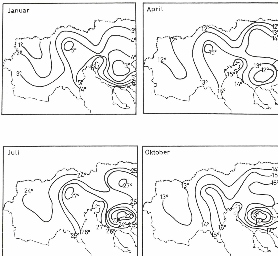
Abb. 4a. Isothermenkurven der Lufttemperatur im Januar, April, Juli und Oktober
