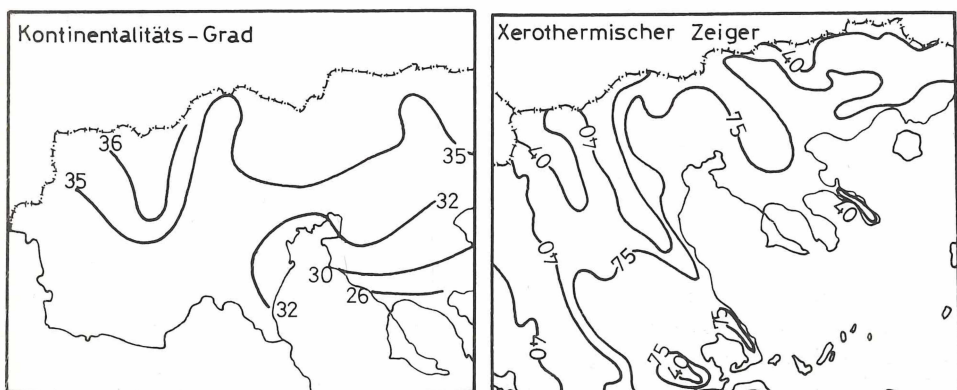
Abb. 4b. Kontinentalitäts-Grad und xerothermischer Zeiger NW-Griechenlands.
