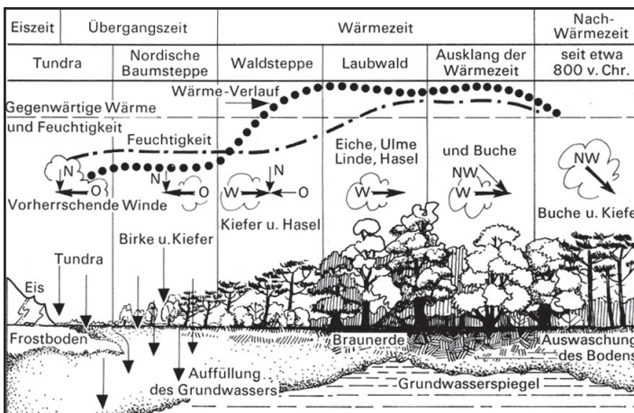
Abb. 2 Schematische Darstellung der Entwicklung des Waldes in der Nacheiszeit in Deutschland: Aus der Tundra der Eiszeit entwickelte sich die nordische Baumsteppe mit Birke und Kiefer, bis dieser die Waldsteppe mit Kiefer und Hasel folgte. Dann folgte ein Laubwald mit Eiche, Ulme, Linde, Hasel usw. bis die Buche sich Richtung Norden langsam etwa gleichzeitig mit der Landwirtschaft um 5000 v. Chr. in Mitteleuropa ausbreitete (BÄRTELS & FUCHS 1976).
