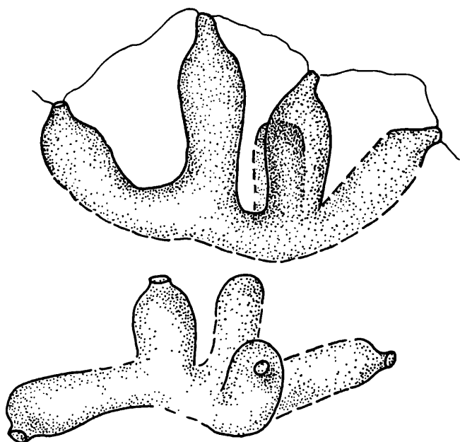
Abb. 1. Seitliche Ansicht der Upogebia operculata Gänge in einer Kalkrotalgenkruste (NHMW 4534); nach einem Formasil-Ausguß gezeichnet. Gangdurchmesser um 12 mm (Tab. 2). Vergleiche Taf. 3, Fig. 5a–b.
