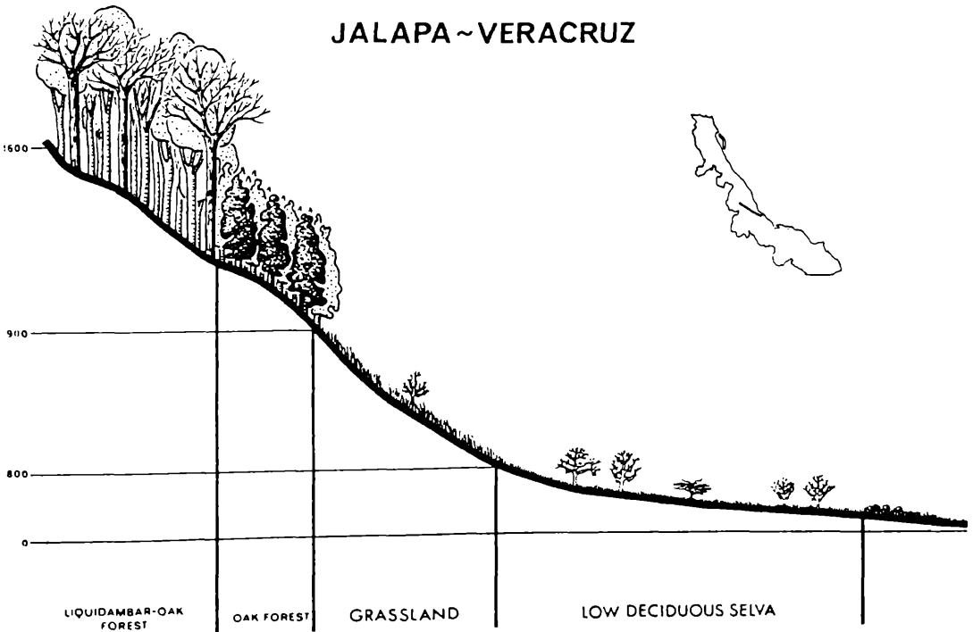
Abb. 15. Vegetationsprofile von der mexikanischen Golfküste (Vera Cruz). Liquidambar-Wald in 900–1600 m. (Nach A. GOMEZ-POMPA, 1973).
