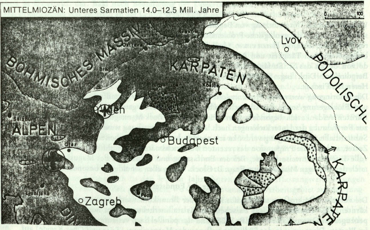
Abb. 2. Zentrale Paratethysküsten (Landmassen grau) (Nach RÖGL & STEININGER 1983).
