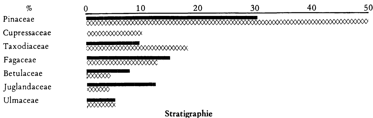
Abb. 9. Prozentueller Anteil der Familien am Pollenspektrum des Unter-Sarmat.
