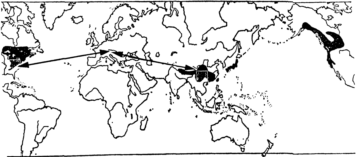
Abb. 17. Rezentareale der Gattung Tsuga (schwarz). Heutige Verbreitung der Tsuga -Fossilien aus dem Unter-Sarmat der Ostalpen. 1. Tsuga canadensis (vel. caroliniana ), 2. Tsuga yunnanensis .
