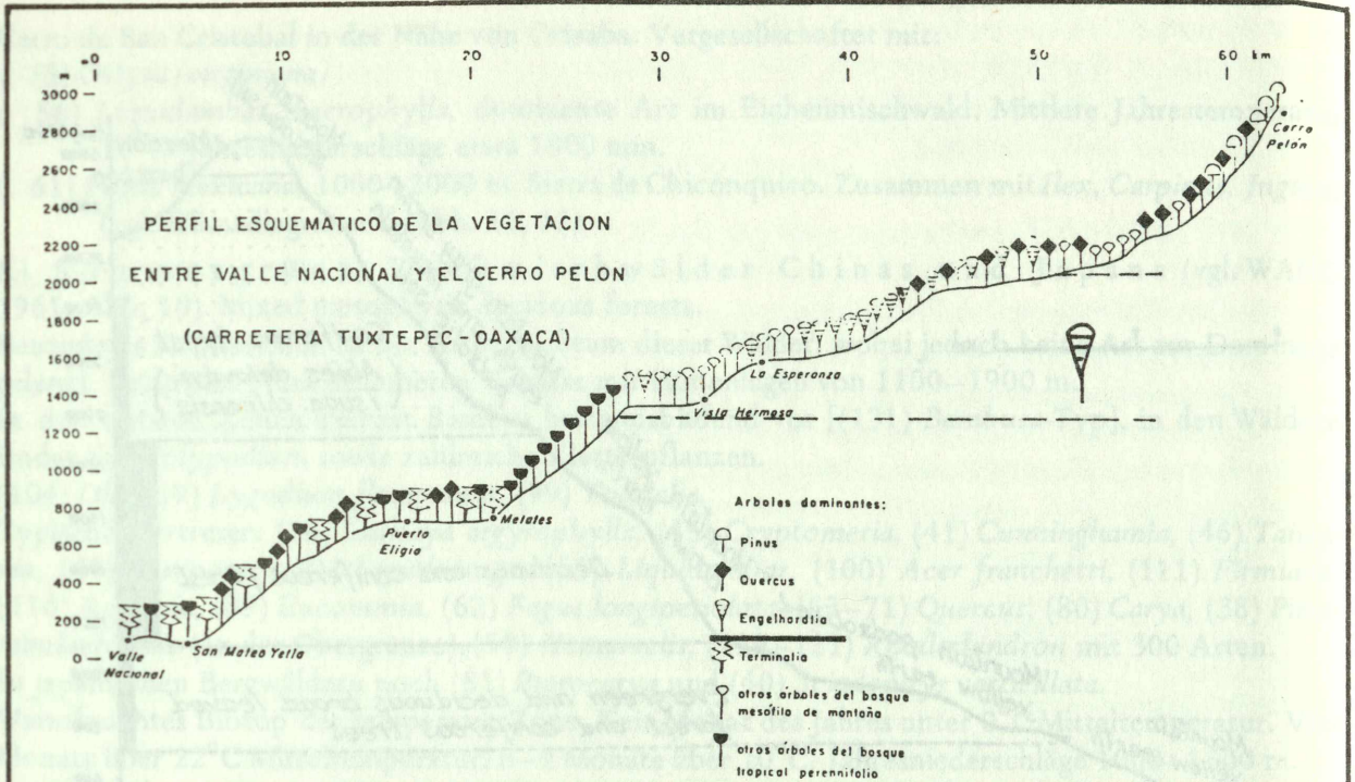
Abb. 14. Vegetationsprofil von Süd-Mexico (Oaxaca, Valle Nacional) mit Engelhardia ( Oreomunnea ) zwischen 1300–2000 m. Das untenstehende Bild zeigt den dichten Bestand des Engelhardia ( Oreomunnea )-Waldes. Aus: RZEDOWSKI & PALACIOS, 1975.
