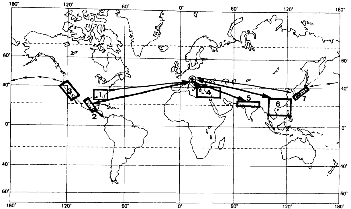
Abb. 16. Areale rezenter Vergleichsformen zu den Pollenfunden des Unter-Sarmat im Lavanttal (Austria).
