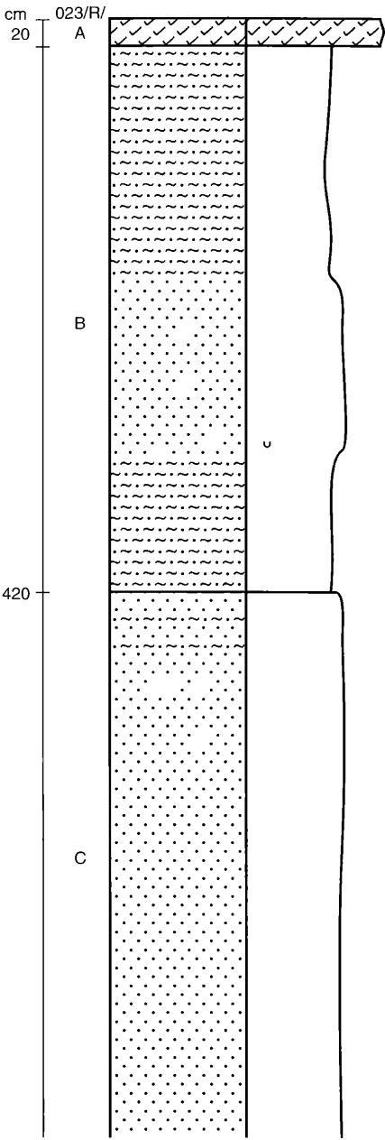
Abb. 19: Profil Obergänserndorf 023/R (Maßstab 1:50)
