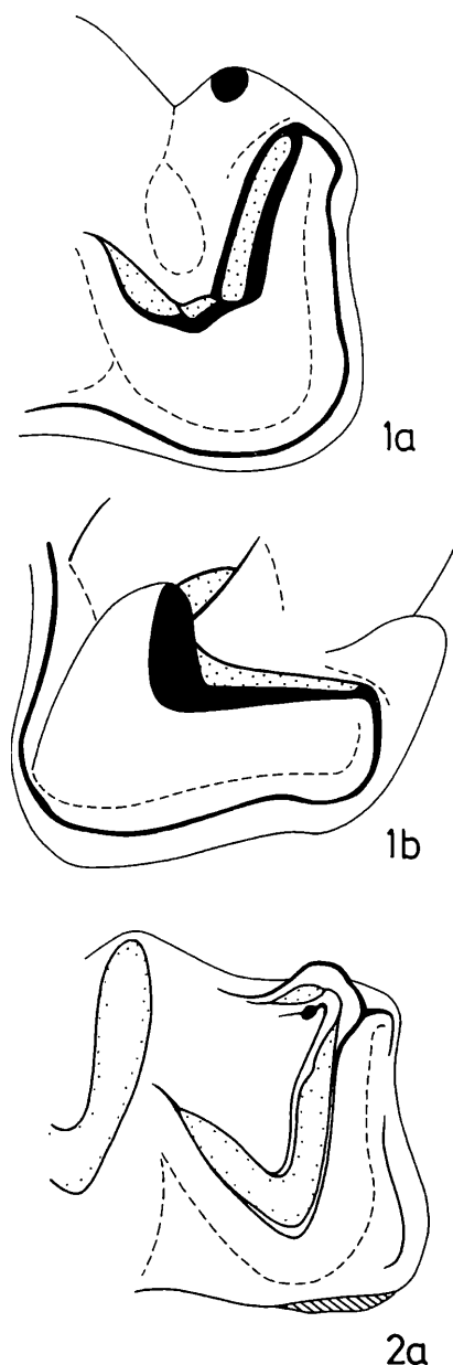
Abb. 8: Talonidabschnitte von zwei M_2 von Dinosorex aus Obergänserndorf
