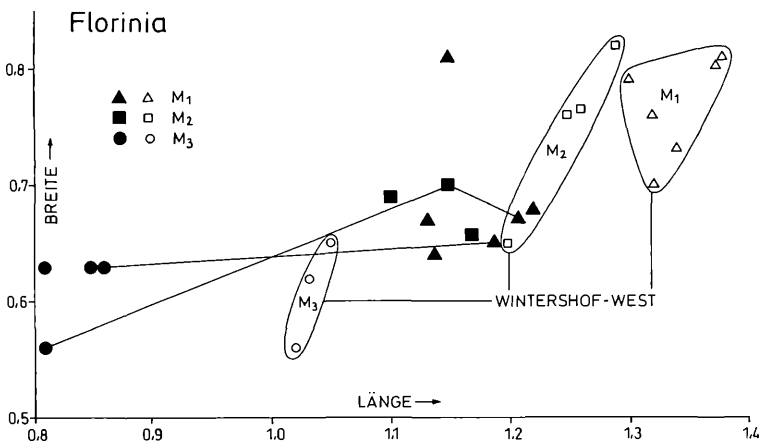
Abb. 11: Längen-Breitendiagramm der M inf. von F. cf. stehlini aus Obergänserndorf im Vergleich zu F. stehlini aus Wintershof-West. Zusammengehörige Molaren sind durch Linien verbunden; Vergleichswerte nach ZIEGLER, 1990
