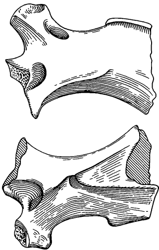
Abb. 4: Humerus-Fragment sin. von Desmanodon cf. antiquus aus Obergänserndorf in Vorder- und Hinteransicht, ca. 6-fach. (NHMW 1997z/0166/25).
