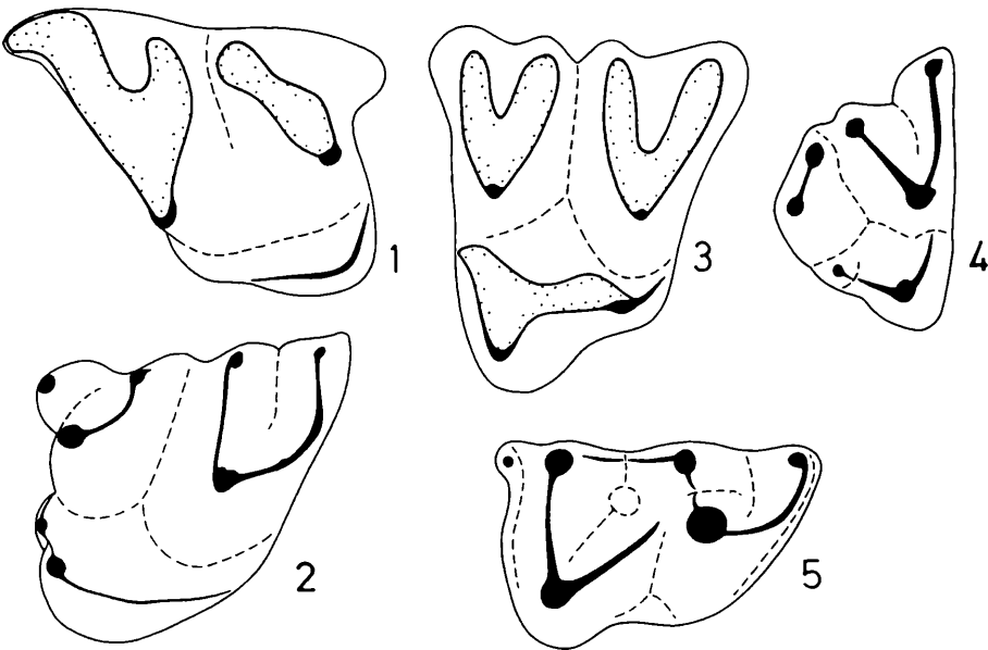
Abb. 3: Schematische Kauflächenbilder der Molaren von Desmanodon cf. antiquus aus Obergänserndorf, ca. 20-fach. Fig. 1: M 1 dext., Fig. 2: M 1 sin., Fig. 3: M 2 sin., Fig. 4: M 3 dext., Fig. 5: M 1 dext. (NHMW 1997z/0166/0002/2, 5, 9, 6 und 15).
