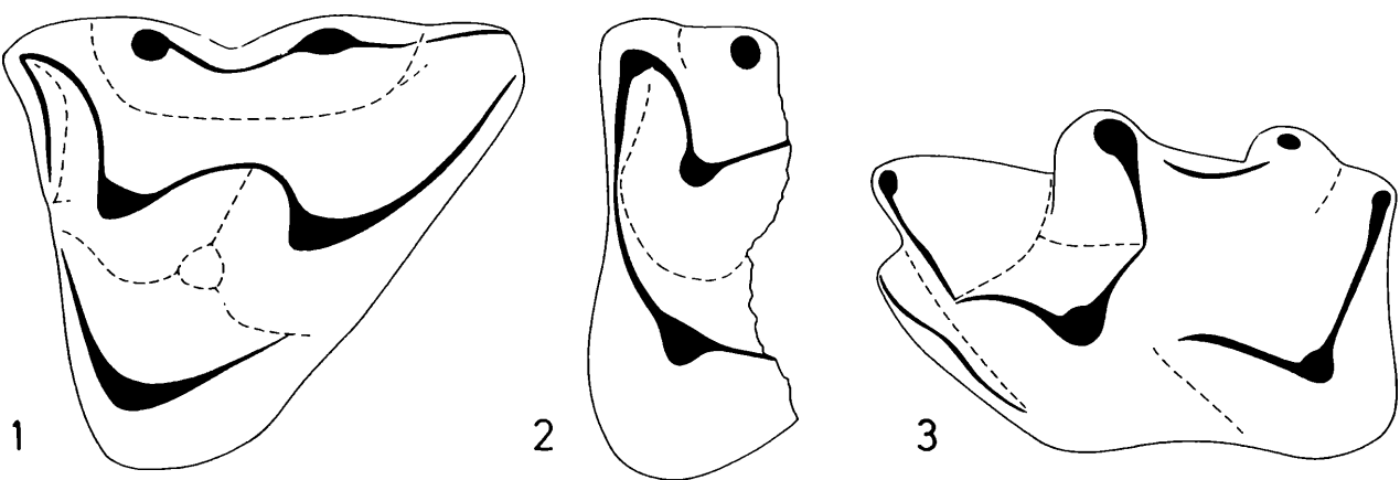
Abb. 14: Amphiperatherium sp. vom Teiritzberg (Fig. 1 und 3) und aus Obergänserndorf (Fig. 2). Fig. 1: M¹ sin.; Fig. 2: M¹-Fragment sin.; Fig. 3: M inf. sin.; NHMW 1997z/0172/0001/851, NHMW 1997z/0172/0002/4, NHMW 1997z/0172/0001/861. Vergrößerung: 30-fach.
