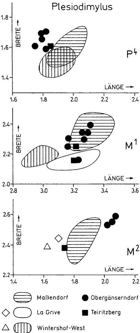
Abb. 6: Längen-Breiten-Diagramm der Oberkieferbackenzähne von Plesiodimylus . Vergleich der Werte von P. cf. bavaricum aus Obergänserndorf und Teiritzberg mit den Werten von P. bavaricum aus Maßendorf, P. chantrei aus La Grive und P. huerzeleri aus Wintershof-West nach SCHÖTZ (1985) sowie von P. helveticum aus Tägersmaustraße-Jonau nach BOLLIGER (1992).
