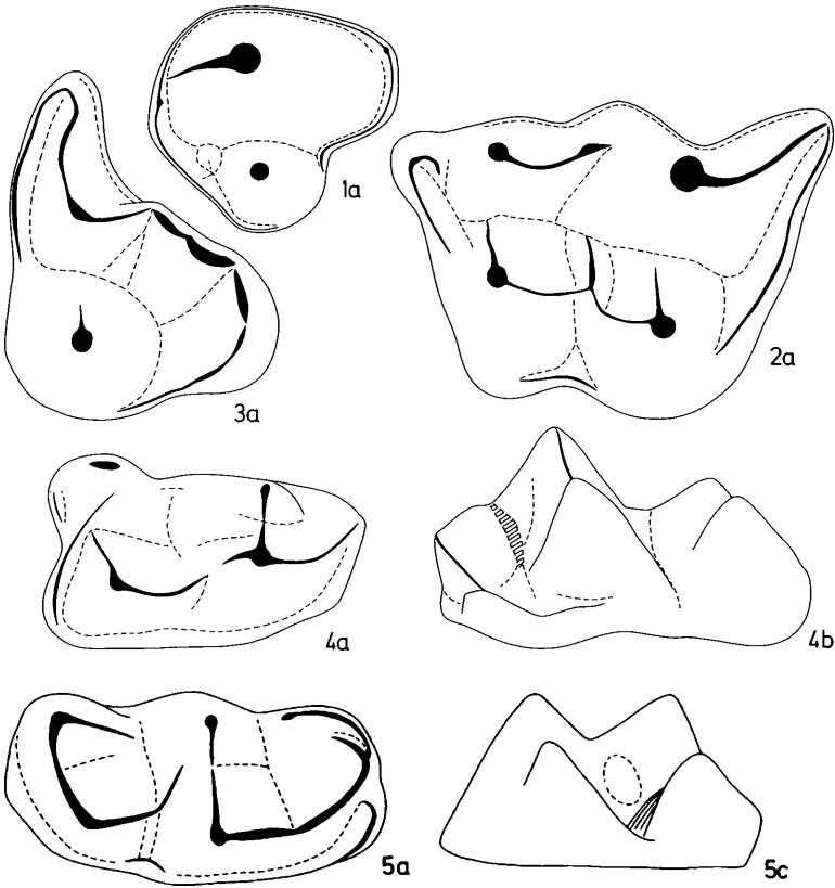
Abb. 5: Schematische Zeichnungen der Backenzähne von Plesiodimylus cf. bavaricum aus Obergänserndorf. Fig. 1: P 4 dext., Fig. 2: M 1 sin., Fig. 3: M 2 sin., Fig. 4: M 1 dext., Fig. 5: M 2 dext. Ansicht: (a) occlusal, (b) lingual, (c) distal (NHMW 1997z/0167/0002/17, 2, 13, 20 und 21), Vergrößerung: alle ca. 18-fach.
