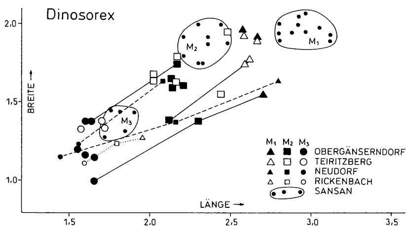
Abb. 9: Längen-Breitendiagramm der M inf. von Dinosorex im Vergleich:
