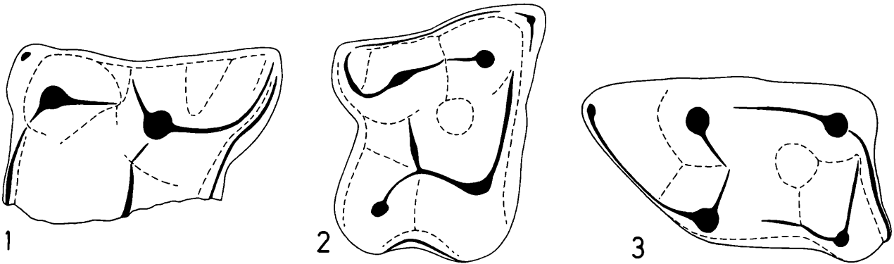
Abb. 13: Mioechinus sp. aus Obergänserndorf Fig. 1: M 1 -Fragment sin.; Fig. 2: M 2 dext.; Fig. 3: M 1 sin. NHMW 1997z/0170/0002/3, NHMW 1997z/0170/0002/2, NHMW 1997z/0170/0002/5. Vergrößerung: 15-fach.
