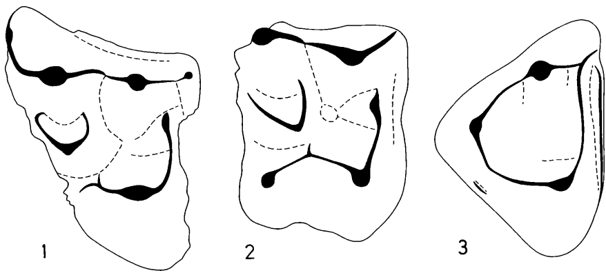
Abb. 12: Galerix sp. vom Teiritzberg. Fig. 1: M 1 -Fragment dext., Fig. 2: M 2 dext., Fig. 3: M 3 dext. Inventarnummern: NHMW 1997z/0171/0001/951, 1997z/0171/0001/952, 1997z/0171/0001/971. Vergrößerung: 20-fach.
