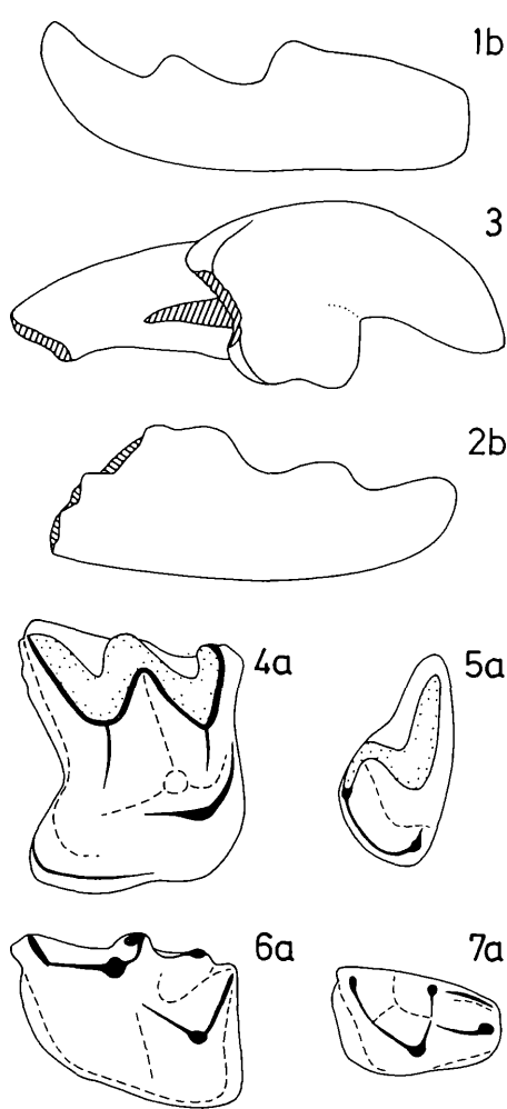
Abb. 10: Florinia cf. stehlini aus Obergänserndorf und vom Teiritzberg. Fig. 1: I inf. sin.; Fig. 2: I inf. Fragment dext.; Fig. 3: I sup. sin.; Fig. 4: M 1 sin.; Fig. 5: M 3 sin.; Fig. 6: M 1 sin.; Fig. 7: M 3 sin.; Ansicht: (a) occlusal, (b) buccal, (c) lingual. NHMW 1997z/0168/0002/3, NHMW 1997z/0168/0002/16, NHMW 1997z/0168/0003/1081, NHMW 1997z/0168/0002/5, NHMW 1997z/0168/0002/11, NHMW 1997z/0168/0002/18, NHMW 1997z/0168/0002/7. Vergrößerung: 25-fach
