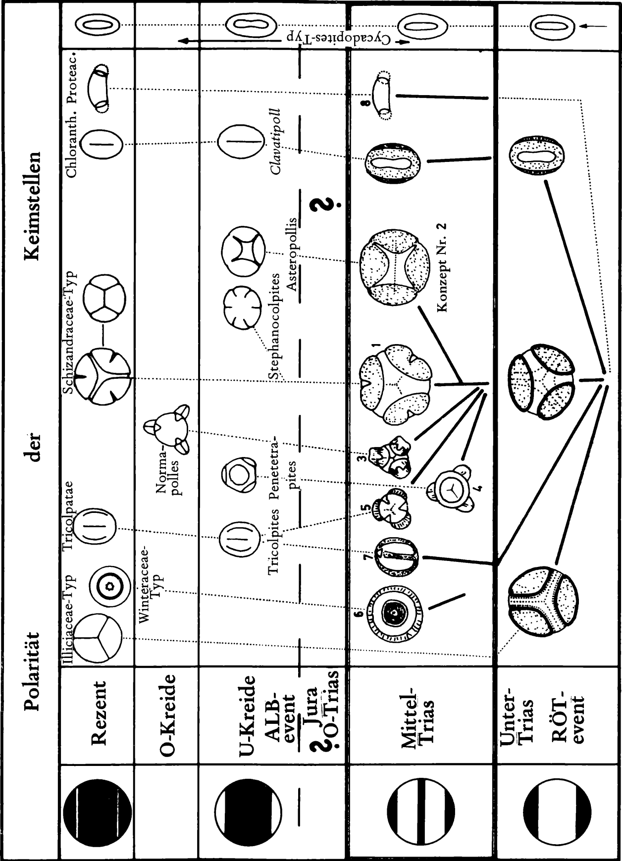
Abb. 9: Die im Text beschriebenen Apertur-Konzepte der Mittel-Trias mit den morphologischen Wurzeln in der Unter-Trias sowie den möglichen morphologischen Entwicklungsformen von Unter-Kreide und Ober-Kreide bis rezent.
