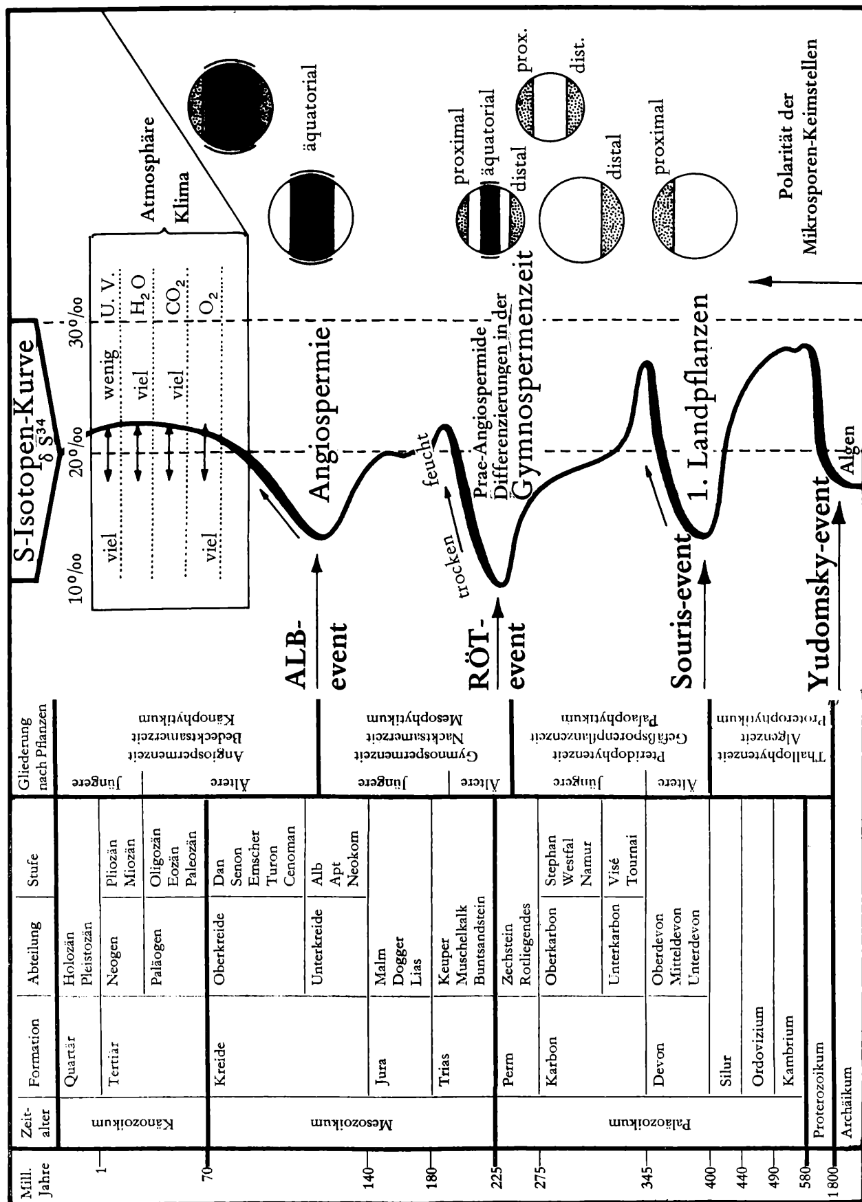
Abb. 6: Abrupte \delta S^{34} Isotopenänderungen im Weltmeer und deren Reflexion auf akzentuierte Evolutionsschritte der Pflanzen im Laufe der Erdgeschichte.
