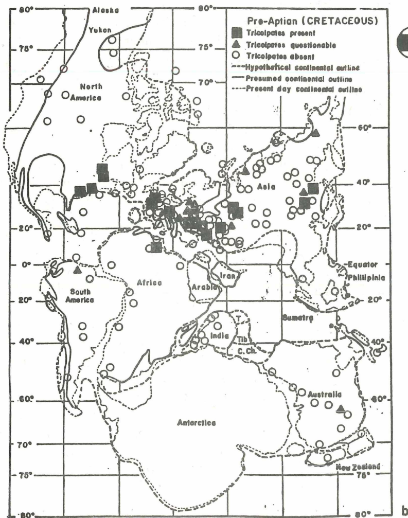
Abb. 7 a. Ozeanöffnungen und \delta S^{34} Alb-event mit folgenden ersten Angiospermenpollen-Fundstellen (nach SRIVASTAVA, 1976 verändert).
