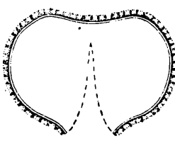
Abb. 2: Mittel-Trias Pollenapertur-Konzept im Vergleich zur rezenten Angiospermenfamilie Schizandraceae (Ziffern-erklärung im Text).
