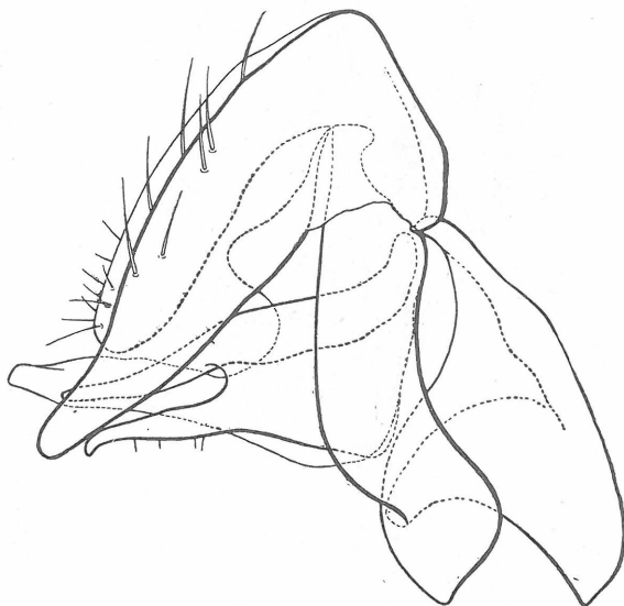
Fig. 2. Leucopis (Leucopis) aphidiperda RONDANI ♂ (Lectotypus): Hypopygium und innerer Kopulationsapparat, Lateralaspekt
