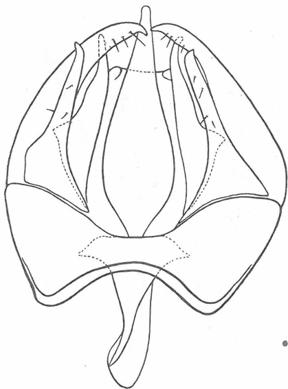
Fig. 1. Leucopis (Leucopis) aphidiperda RONDANI ♂ (Lectotypus): Hypopygium und innerer Kopulationsapparat, Ventralaspekt
