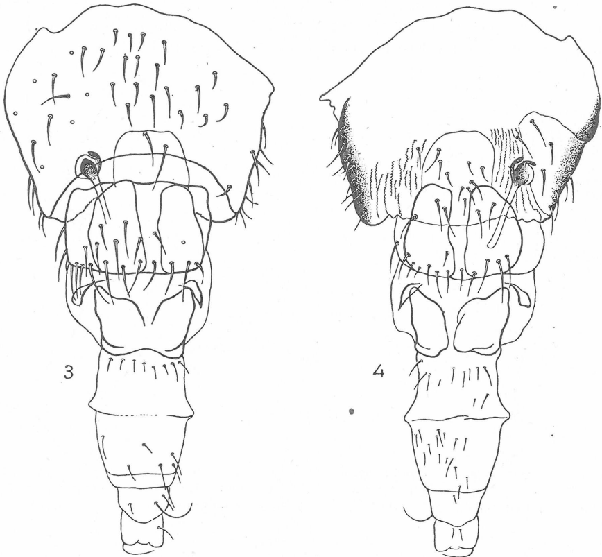
Leucopis (Leucopis) aphidivora RONDANI ♀ (Lectotypus): Fig. 3. Legrohr in Dorsalansicht — Fig. 4. Legrohr in Ventralansicht
