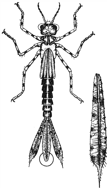
Fig. 1. Platycnemis pennipes (PALLAS): Larve (nach POPOVA, 1953). (Besonders zu beachten ist das mittlere Analblatt; Kreis von mir eingezeichnet.)
