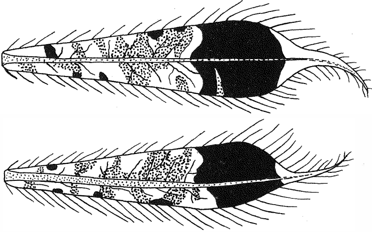
Fig. 3. Platycnemis pennipes (PALLAS): Analanhänge einer Larve im letzten Stadium (Original). Fundort: Etang de Commelles bei Chantilly (Oise). (Oben: mittleres Analblatt — unten: linkes äußeres Analblatt)
