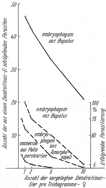
Fig. 2. Parasitierung und Nachkommenzahl in Abhängigkeit von der Anzahl vorgelegter Dendrolimus pini -Eier
