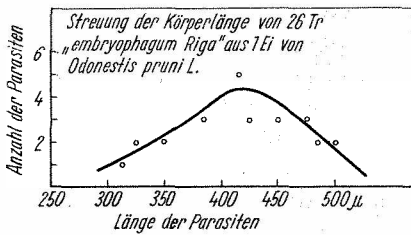
Fig. 3. Geschwister aus dem gleichen Wirtsei besitzen meist sehr unterschiedliche Körpergröße
