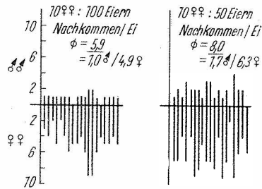
Fig. 6. Parasitendichte und Sexualindex bei Tr. semblidis AURIVILLUS (Stamm 15) in jeweils einem Arctia -Ei
