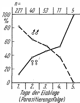
Fig. 9. Veränderung des Sexualindex bei Tr. embryophagum HARTIG (Stamm 35) in Beziehung zur Parasitierungsfolge in Arctia caja LINNÉ
