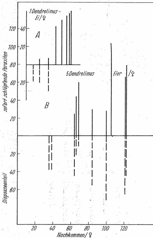
Fig. 15. Diapause und Parasitendichte von Tr. embryophagum HARTIG (Stamm 35) bei Vorlage von je 1 beziehungsweise je 5 Dendrolimus -Eiern/φ (20–24 °C, 60 bis 80%, 18/6)
