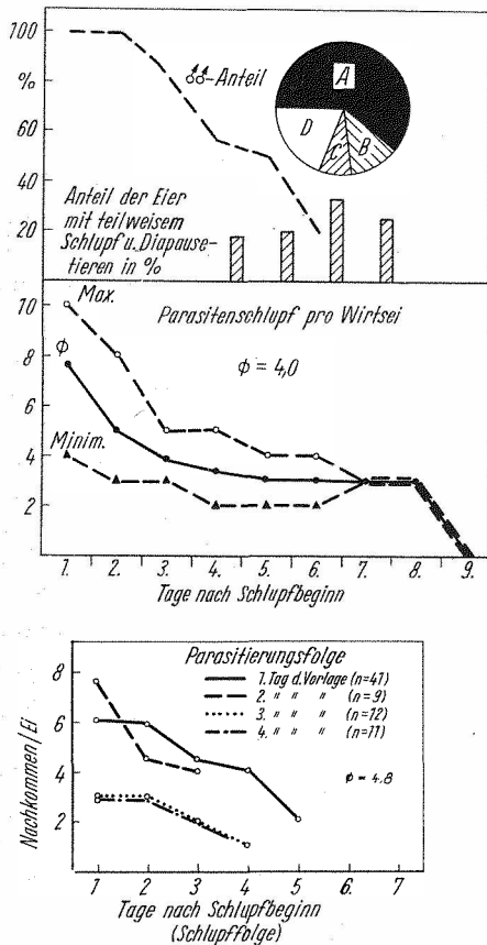
Fig. 10. Parasitierungsdichte und endogene Diapause bei Tr. embryophagum HARTIG (Stamm 35) in Abhängigkeit von der — hier nicht unterschiedenen — Parasitierungs- und Schlupffolge (21 °C, 65%, 18/6; A—D siehe Text)
