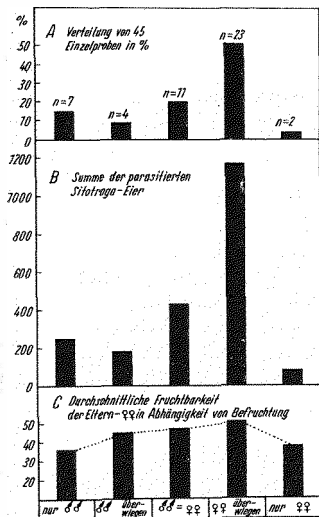
Fig. 8. Verteilung der Geschlechter bei einer Fruchtbarkeitsanalyse von Tr. evanescens WESTWOOD (Stamm 2) und einem Sexualindex von 37/63 der Elterngeneration
