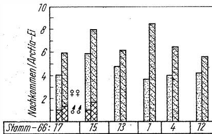
Fig. 5. Beeinflussung der Parasitendichte durch hohes oder niederes Angebot von Wirtseiern bei verschiedenen Trichogramma -Stämmen (erste Säule = 100 Arctia -Eier: 10 ♀♀; zweite Säule = 50 Arctia -Eier: 10 ♀♀)
