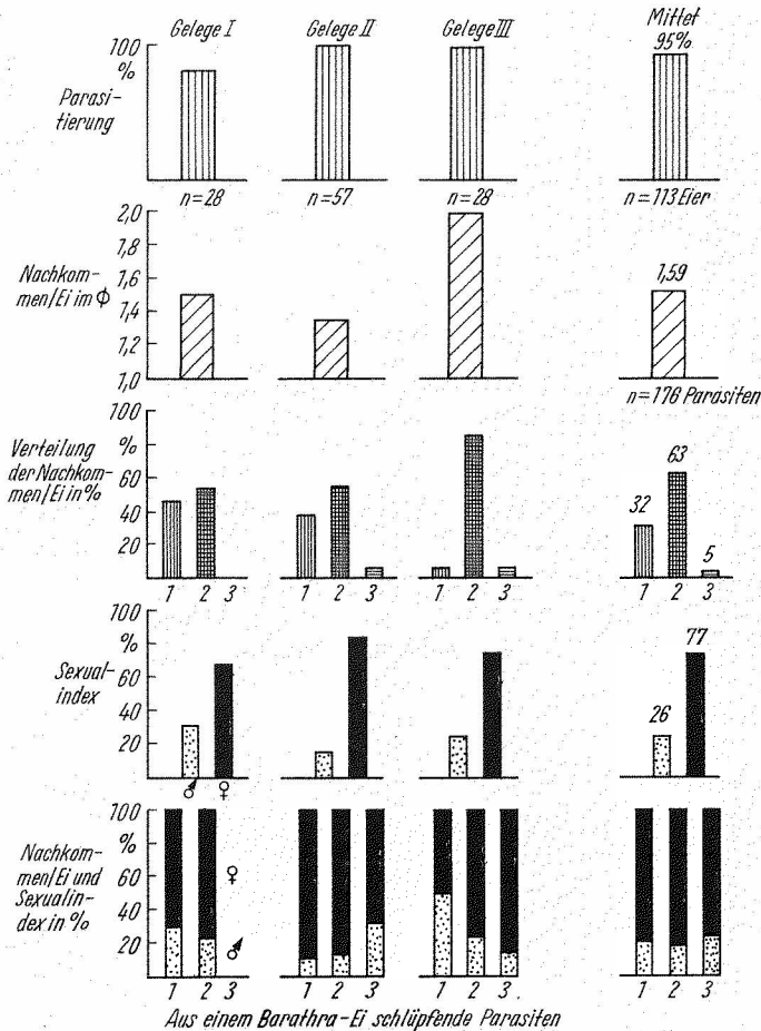
Fig. 7. Schlupfanalyse einiger im Freiland durch Tr. evanescens WESTWOOD parasitierter Gelege von Barathra brassicae LINNÉ (Ausgangsmaterial für Stammzucht Nr. 36)
