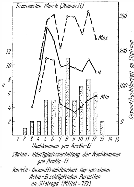
Fig. 12. Die optimale Parasitierungsdichte im Arctia -Ei, gemessen an der Gesamtfertbarkeit der jeweils aus einem Ei schlüpfenden Parasiten (21–24°C, 60–80%, 18/6)
