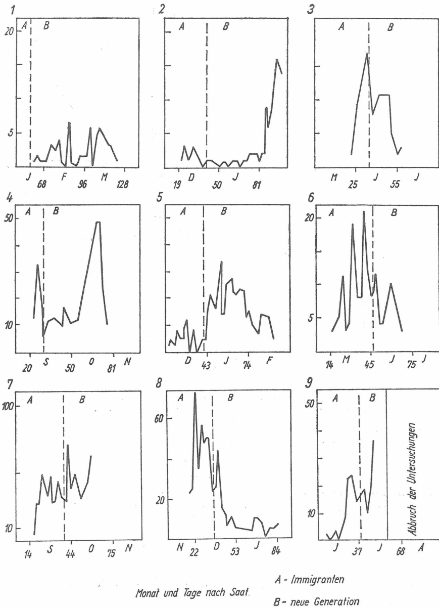
Fig. 1: Abundanzdynamik von Diabrotica balteata LEC. in 9 Bohnensaat
