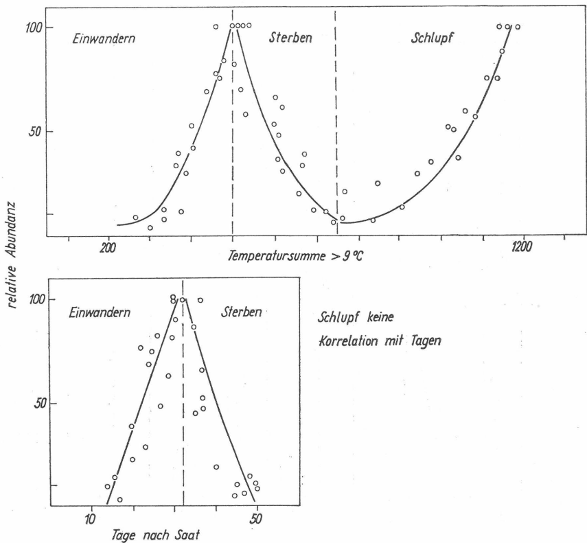
Fig. 2: Abundanzdynamik von Diabrotica balteata LEC. in Bohnenbeständen in Abhängigkeit vom Pflanzenalter und der Temperatursumme > 9^{\circ}\text{C}
