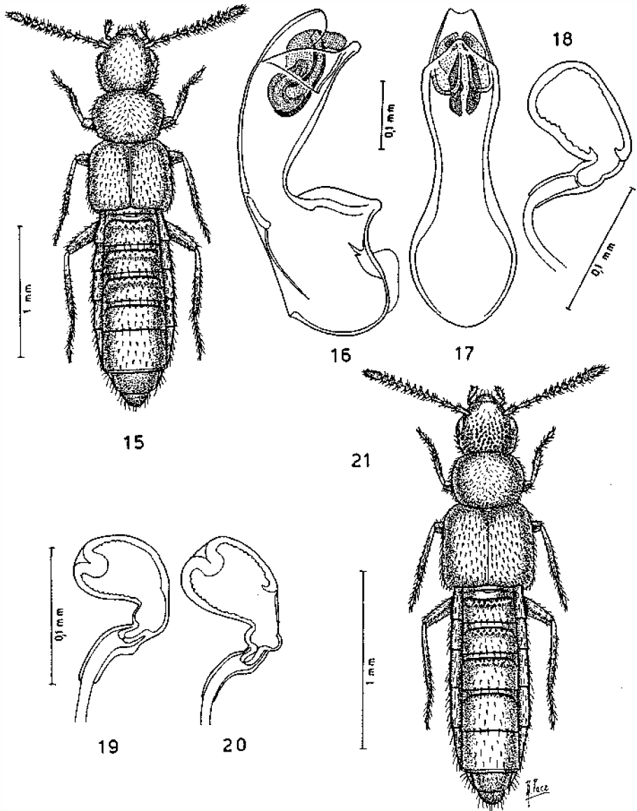
Figg. 15-21: Habitus, eedeago in visione laterale e ventrale e spermateca. 15-18. Leptusa (Akratopisalia) xianensis sp. n., Shaanxi: Qinling Shan; 19-21: Leptusa (Akratopisalia) quinlingensis sp. n., Shaanxi: Qinling Shan (19. holotypus; 20. paratypus).
