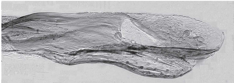
Fig. 15: Stauronematus saliciphilus sp. n. Penisvalve (detail).
