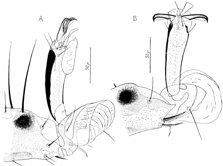
Fig. 13. Schienenende und Tarsus von Myrsidea cornicis (Deeger) (Menoponidae, Amblycera), A — vom rechten Hinterbein, Tarsus in Seitenansicht, B — vom linken Mittelbein, Tarsus in Dorsalansicht
