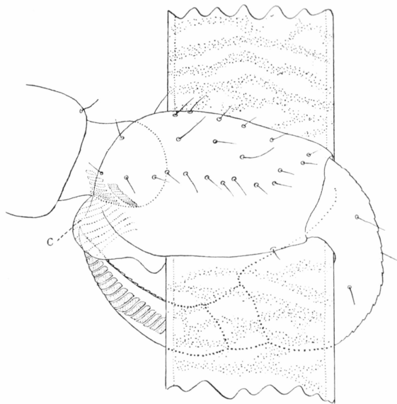
Fig. 5. Rechtes Mittelbein von Gyropus ovalis Nitzsch mit gelockertem Verschluss, ein Haar umklammernd. c — wie in Fig. 3
