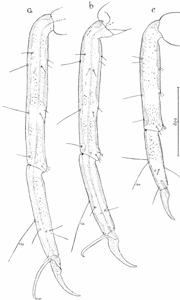
Fig. 14. Linkes Hinter- (a), Mittel- (b) und Vorderbein (c) von Haematomyzus elephantis Piaget (vom indischen Elefanten), a und b von der Dorsalseite, c von der Ventralseite. Die Zahlen an den Borsten geben ihre Längen in Mikron an
