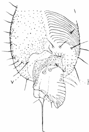
Fig. 11. Schienenende und Tarsus vom rechten Hinterbein von Gliricola porcelli (Linné) (Weibchen). Ansicht schräg von innen, außen und von der Spitze. Bezeichnungen wie in Fig. 9 und 10
