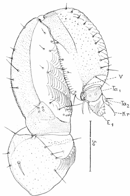
Fig. 8. Linkes Hinterbein eines Weibchens von Gliricola porcelli . Ansicht von vorn. v — Tarsifer anterior, sonstige Bezeichnungen wie in Fig. 1
