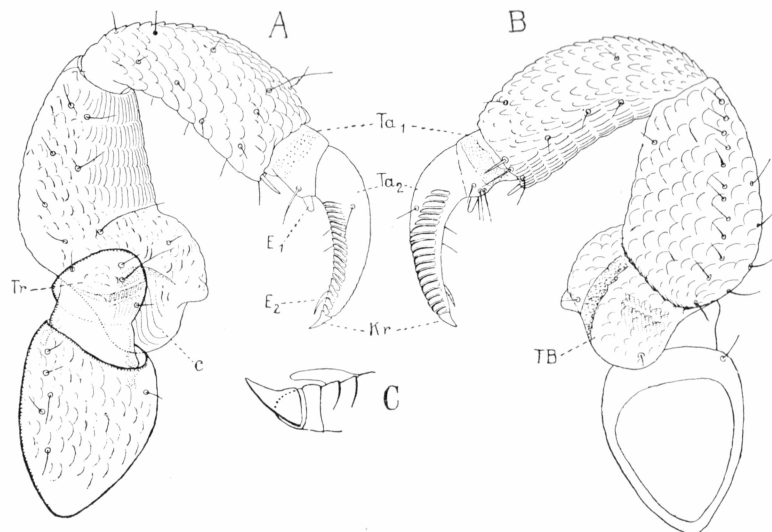
Fig. 1. Linkes Hinterbein eines Männchens von Gyropus ovalis Nitzsch. A — Ansicht von vorn, B — Ansicht von hinten (das Bein ist senkrecht zur Körperachse ausgestreckt gedacht), C — Tarsenspitze mit Krallen, von vorn. Ta 1 — erstes, Ta 2 — zweites Tarsenglied, Kr — Krallen, E 1 — Euplantula des ersten, E 2 — Euplantula des zweiten Tarsengliedes, TB — Tenakulum-Buckel, Tr — Trochanter, c — Rillen auf der Innenwand des Tenakulum-Buckels
