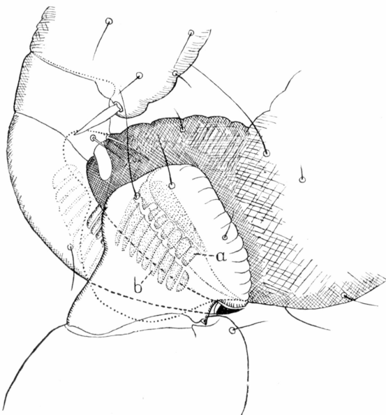
Fig. 4. Tenakulum des linken Hinterbeines eines Männchens von Gyropus ovalis Nitzsch in fast geschlossener Klammerstellung bei der Ansicht von vorn (vgl. Text zu Fig. 1). Bezeichnungen vgl. Fig. 3
