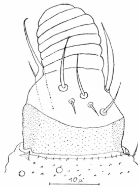
Fig. 12. Rechter Vorder-tarsus des 3. Nymphenstadiums von Gliricola porcelli (Linné). Ansicht von innen
