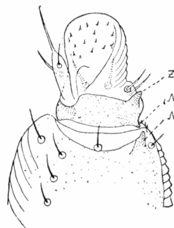
Fig. 9. Schienenende und Tarsus vom linken Hinterbein eines Weibchens von Gliricola porcelli (Linné). Ansicht von schräg vorn und außen. v — Tarsifer anterior, v' — Gelenkvorsprung des Basitarsus, z — Zahn des Basitarsus
