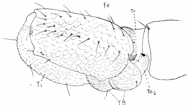
Fig. 2. Linkes Mittelbein eines Weibchens von Gyropus ovalis Nitzsch in Klammerstellung mit gelockertem Verschuß. Fe — Schenkel, Ti — Schiene, übrige Bezeichnungen wie in Fig. 1
