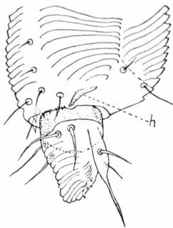
Fig. 10. Schienenende und Tarsus vom rechten Hinterbein von Gliricola porcelli (Linné). Ansicht von hinten. h — Tarsifer posterior
