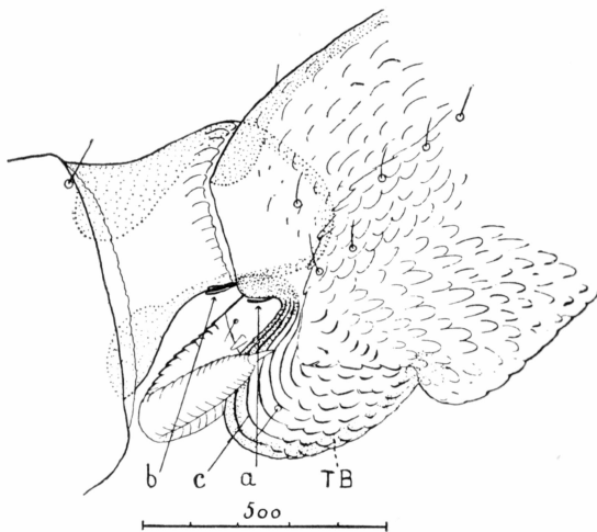
Fig. 3. Tenakulum des rechten Mittelbeines von Gyropus ovalis Nitzsch. Dorsalansicht schräg von vorn. Das Bein befindet sich in Klammerstellung, das 2. Tarsenglied gelockert im Tenakulum-Sattel. a — die femorale, b — die trochanterale Kerben-Reihe, c — Kerben auf der Innenwand des Tenakulum-Buckels
