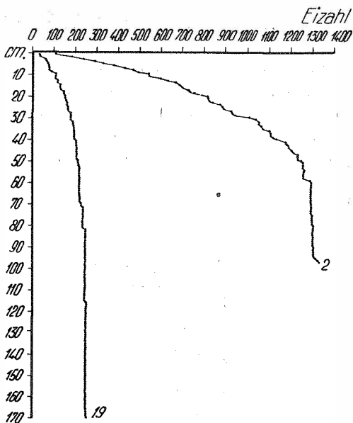
Fig. 5. Summierte Eizahlen von Zweig Nr. 2 und Nr. 19
