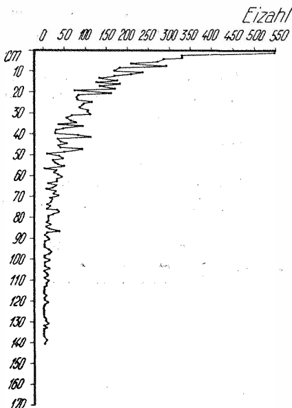
Fig. 3. Gesamteiverteilung auf 10 Zweigen bei Baum Nr. 1
