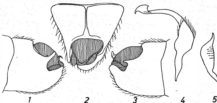
Fig. 1—5. Phytocoris pilifer Reut., Genitalien des Männchens. — Fig. 1. Genitalsegment von links (22,5 x). — Fig. 2. Dasselbe von oben (22,5 x). — Fig. 3. Dasselbe von rechts (22,5 x). — Fig. 4. Linke Paramere seitlich (120 x). — Fig. 5. Rechte Paramere seitlich (120 x)
