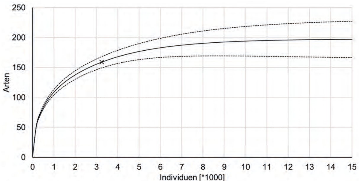
Fig. 3: Kombinierte Rarefaction- und Extrapolationskurve der erfassten Wildbienen. x Beobachteter Wert. – Inter- bzw. Extrapolation. - - 95 %-Konfidenzintervall.
