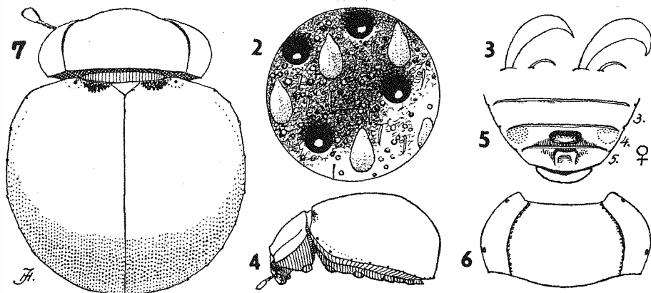
Fig. 2—7. Notiophygus ignoratus n. sp. Fig. 2. Elytrale Sculptur, Haartyp 1c. — Fig. 3. Haare seitlich. — Fig. 4. Seitenansicht. — Fig. 5. Sternite ♀. — Fig. 6. Pronotum unverkürzt. — Fig. 7. Umriß
