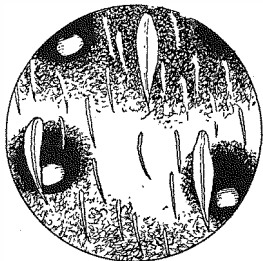
Fig. 1. Notiophygus umdalanus n. sp. Sculpturbild
