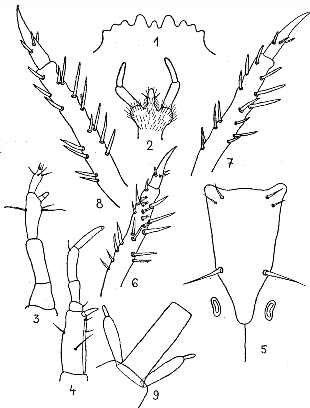
Fig. 1—9. Larve von Quedius vexans Eppelsheim. 1. Vorderrand des Clypeus. — 2. Labium. — 3. Fühler. — 4. Maxille. — 5. Gula mit den Einlenkungsstellen des Tentoriums. — 6, 7, 8. Vorder-, Mittel- und Hinterschiene. — 9. Analpseudopod und die Urogomphen
