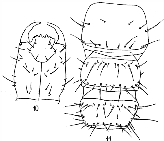
Fig. 10—11. Larve von Quedius vexans Eppelsheim. 10. Kopf von oben mit Chaetotaxie. — 11. Thorakalsegmente mit Chaetotaxie
