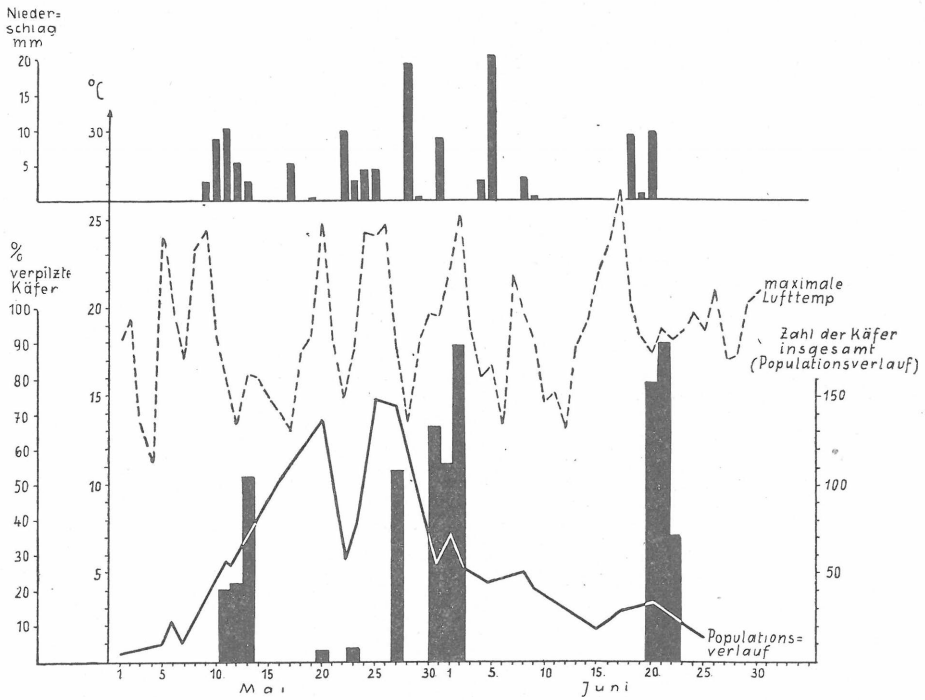
Fig. 3. Auftreten verpilzter Leinerdlöhe in Abhängigkeit vom Populationsverlauf, der Temperatur und den Niederschlägen. Aschersleben 1958. Wasserschalenfänge
