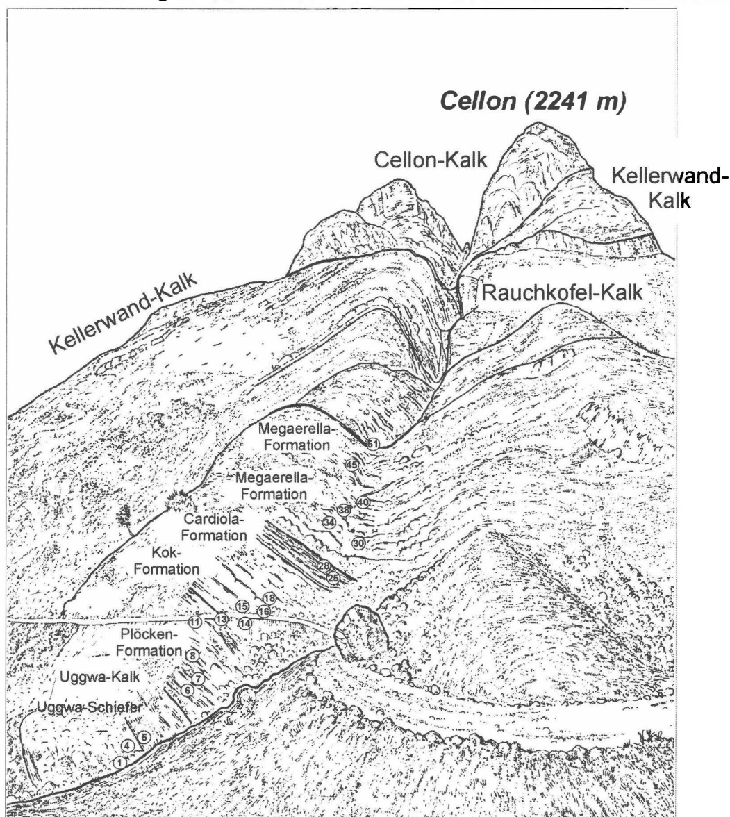
Abb.3: Die Cellonetta-Lawinenrinne mit ihren lithostratigraphischen Einheiten. Die Nummern korrespondieren mit den im Text erwähnten Probennummern (verändert nach SCHÖNLAUB 1991).
