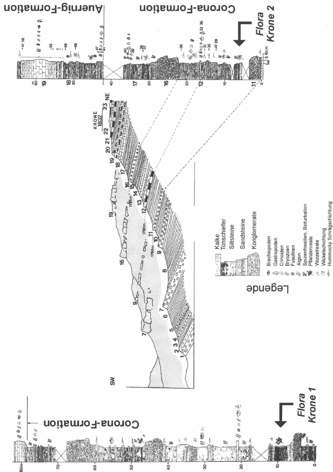
Abb.8: Profile durch die Westseite der Krone mit dem Pflanzenfossilfundpunkt „Flora Krone 1“ bei Seehöhe 1760 m und durch die Südseite der Krone mit Position der Megaflora „Flora Krone 2“ bei Seehöhe 1770 m. Verändert nach KRAINER (1990) und FRITZ & KRAINER (1993) bzw. GEYER (1897). Beachte Lage des Fossilfundpunktes „Flora Krone 2“ innerhalb der Schicht 11 im Geländeprofil von GEYER.
