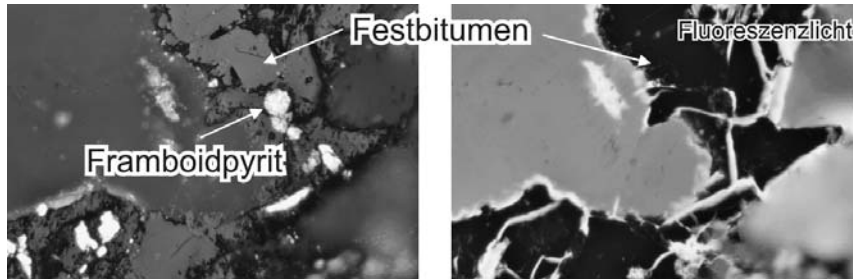
Abb. 4: Festbitumen und Pyrit im Anschliffbild (Normal- und Fluoreszenzlicht). Die Bildlänge beträgt 0,22 mm
