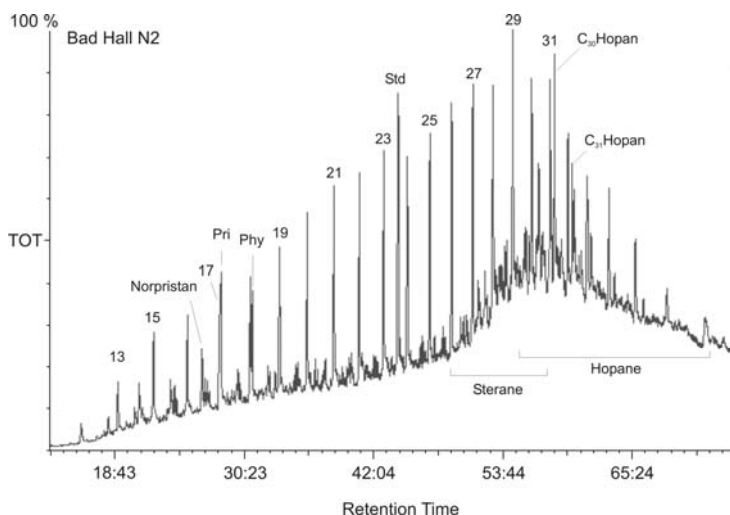
Abb. 6: Gaschromatogramm der Aliphatenfraktion des Festbitumens (Bohrung BH N2)
