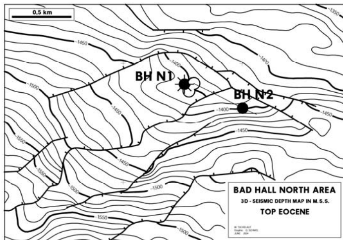
Abb. 1: Bad Hall Nord - Strukturkarte Top Eozän
