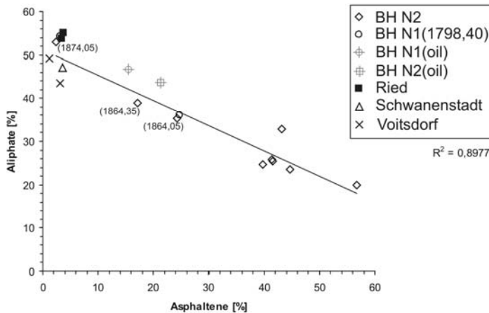
Abb. 5: Plot der Asphaltengehalte gegen die Aliphatgehalte.
