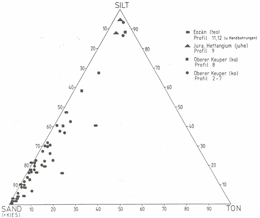
Abb. 13: Konzentrationsdreieck Sand (+ Kies)/Silt/Ton der Rhät-, Lias- und Tertiärproben (aus HESSLER 1979)
