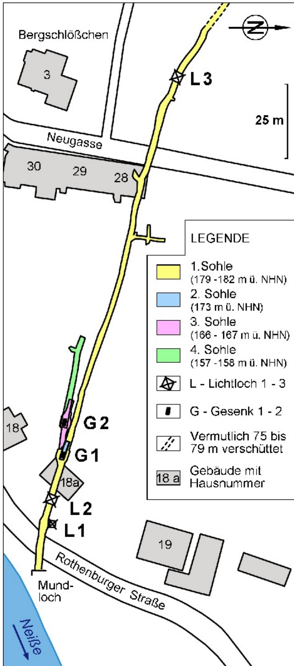
Karte 1 Bergwerk Goldgrube von Görlitz mit Grubenriss und Längsprofil (S. 105) Stand 03/2013. Riss und Profil wurden nach der Sanierungsdokumentation (OBA-FG: KLÖDEN & GELBRICHT 2012), der topographischen Karte TK 10 (Blatt Görlitz) und eigenen Befahrungen erstellt. Anmerkung: Die Lichtlöcher 1–3 sind inzwischen verwahrt.
