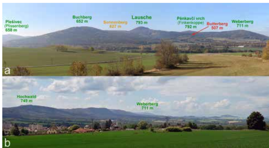
Abb. 2a: Blick von Norden auf die fast 200 m hohe Steilstufe des Zittauer Gebirges zwischen Jonsdorf und Waltersdorf (im Foto rechts). Die kreidezeitlichen Sandsteine bilden ein angehobenes Plateau (z. B. sichtbar am Sonnenberg, gelb), welches nochmals von Phonolith-Vulkankuppen (grün) überragt wird (bei der Lausche zusätzlich mit Basaltsockel!). Am Fuß der Steilstufe verläuft die Lausitzer Überschiebung, an der im Vordergrund die granitischen Gesteine (rot, z. B. am Butterberg) des Lausitzer Blocks angrenzen. Foto: O. Tietz
