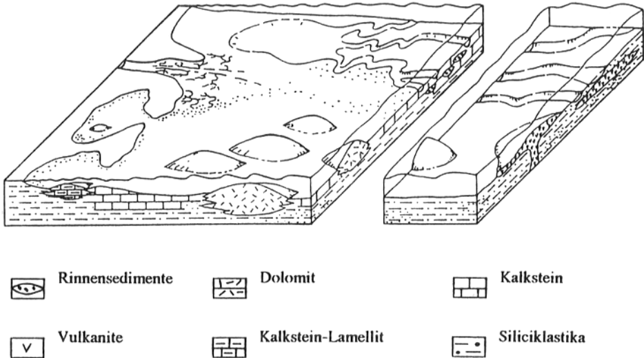
Abb. 3 Faziesmodell des höheren Unterkambriums im Görlitzer Raum (Elicki & Schneider 1992)
