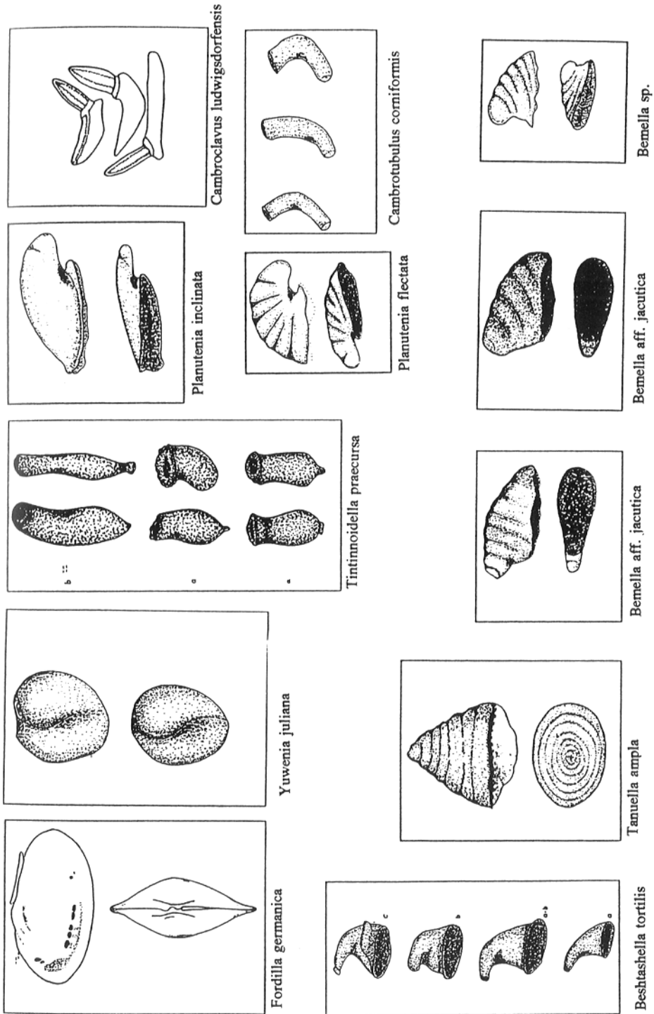
Abb. 4 - Ausgewählte Mikrofossilien (Bruch Ludwigsdorf; Größe 0,3 - 7 mm)
