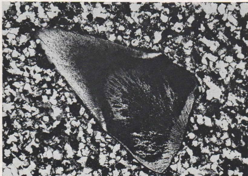
Tafel 2, Bild 3: Gleiche Aufnahme bei gekreuzten Polarisatoren.
