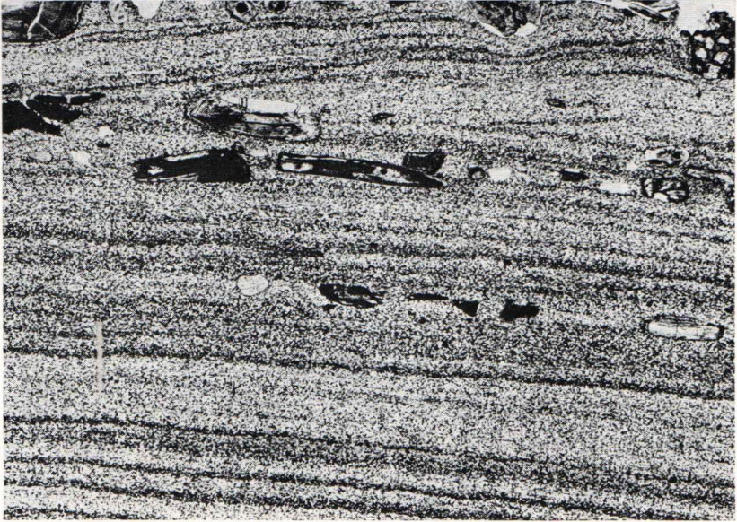
Tafel 3, Bild 4: Rhät-Bonebed, Baugrube Commerzbank Bielefeld, Dünnschliff, Vergrößerung 7,5fach, polarisiertes Licht ohne Analysator, in Schichtebene eingeregelt Bonebed-Bestandteile (Wirbeltierreste, grobe Quarzkörner), Feinschichtung im Feinsandstein.
