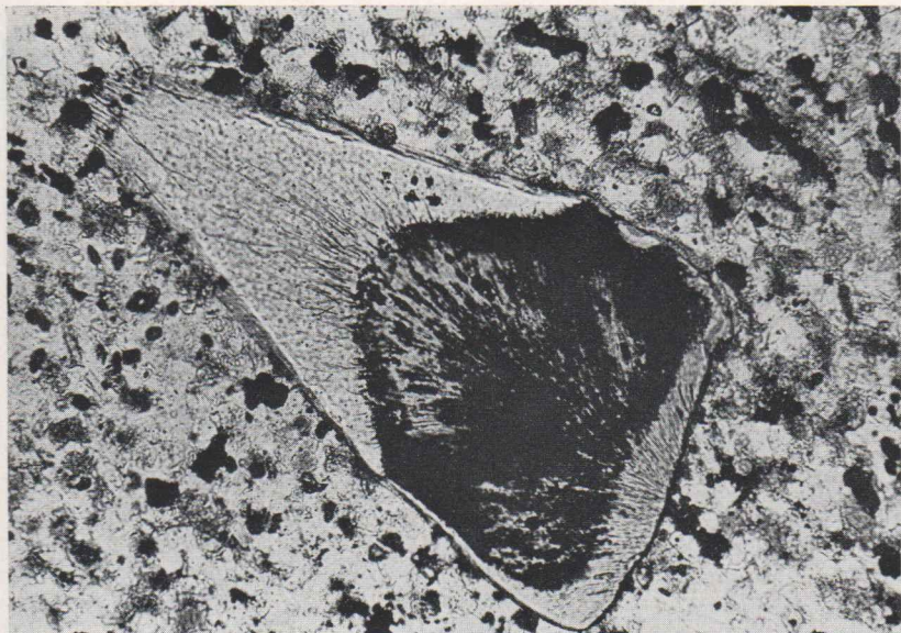
Tafel 2, Bild 2: Rhät-Bonebed, Baugrube Commerzbank Bielefeld, Dünnschliff, Vergrößerung 128fach, polarisiertes Licht ohne Analysator, Schnitt durch Kegelzähnen Saurichthys acuminatus AG. im Feinsandstein.
