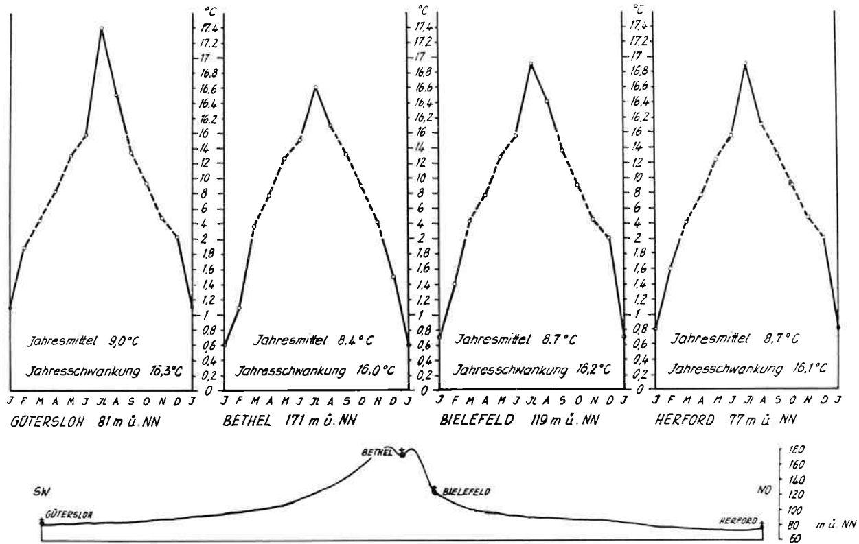
Abb. 1 Profil Gütersloh - Herford (Klimawerte 1881-1930 nach Klimakunde des Dt. Reiches, Bd. I, Berlin 1939)
