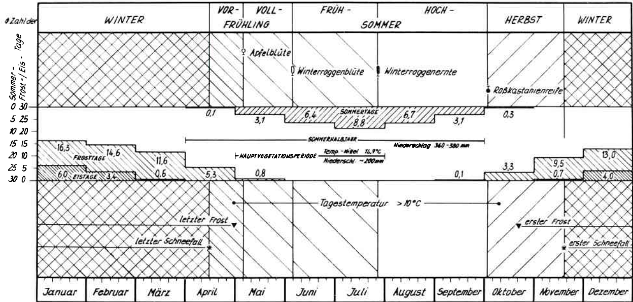
Abb. 2: Phänologisches Diagramm für Herford
