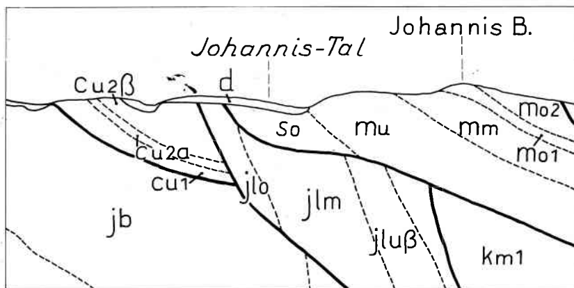
Abbildung 2: Geologisches Profil in der Linie Bahnhof Brackwede - Johannis-Berg (Bielefelder Paß) nach Geol. Kt. Preußen 1:25 000, Blatt 2149 Bielefeld (Lfg. 256), Berlin 1926.
