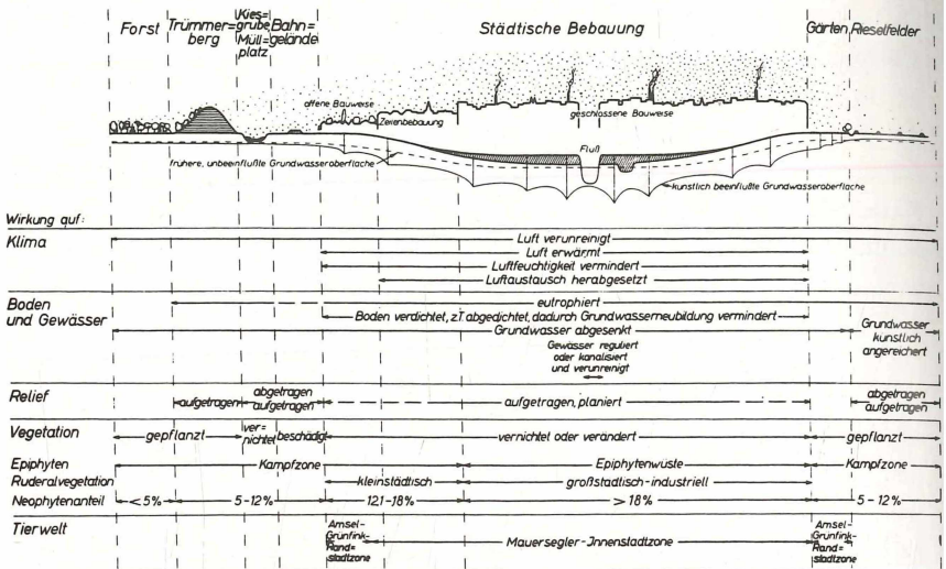
Abb. 2: Veränderungen der Biosphäre in einer Großstadt (nach SUKOPP)
