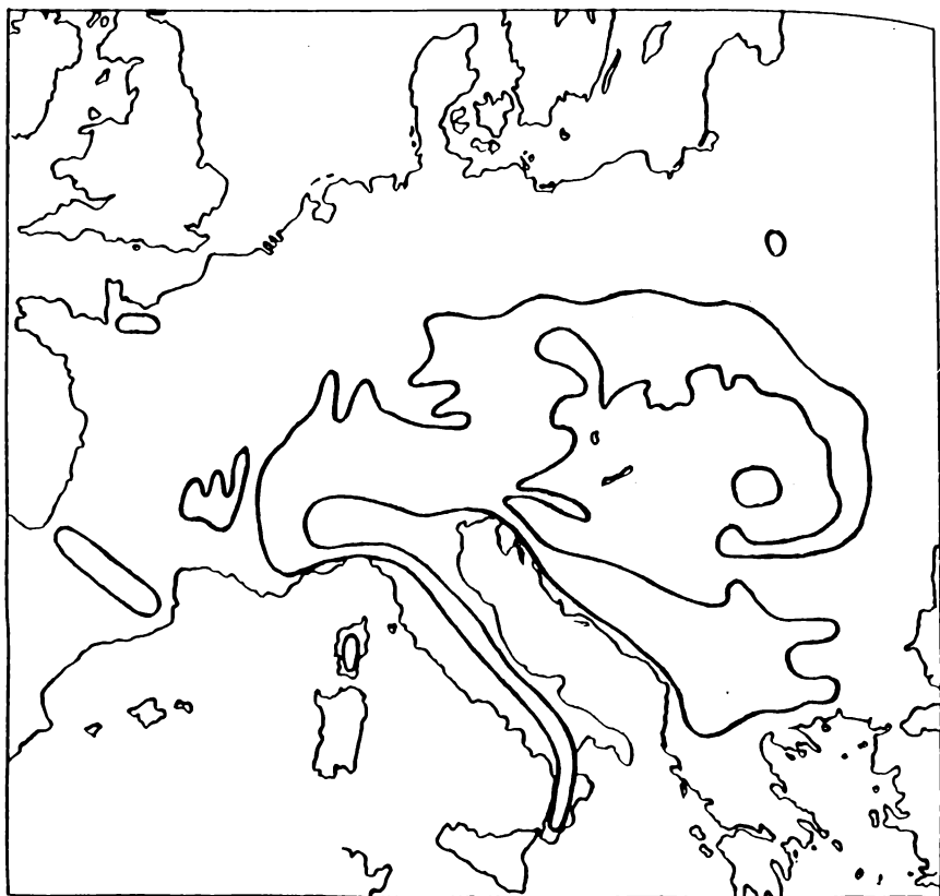
Abb. 3: Ursprüngliches heutiges Areal der Weißtanne in Europa. Nach MATTFELD aus SUESSENGUTH (1936).
