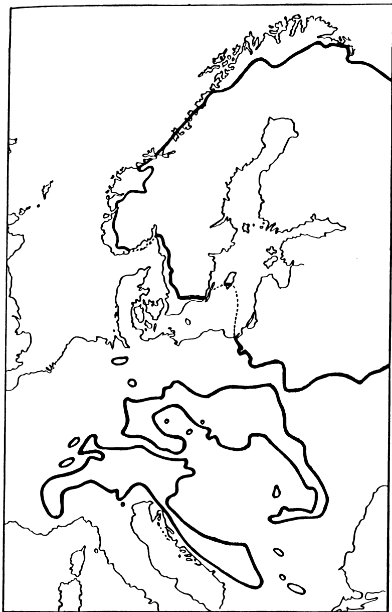
Abb. 2: Ursprüngliches heutiges Areal der Fichte in Europa.
