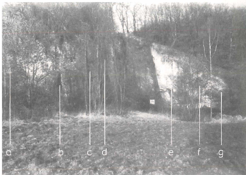
Abb. 3: Naturdenkmal aufgelassener Steinbruch Imkamp am Große Bokermann, Bielefeld Senne. a liegender Bereich des Hyphantoceras Event, b Mergellage M_{Echen} , c Influafter Lage, d Mergellage M_E , Grenze zwischen der Mytiloides striatoconcentricus Zone (links) und der Inoceramus costellatus Zone (rechts), e Tuff T_{D1} und begleitende Mergellage, f Inoceramus costellatus / Sternotaxis plana Event, g laminierte Lage, Grenze zwischen Ober-Turon (links) und Mittel-Turon (rechts).
