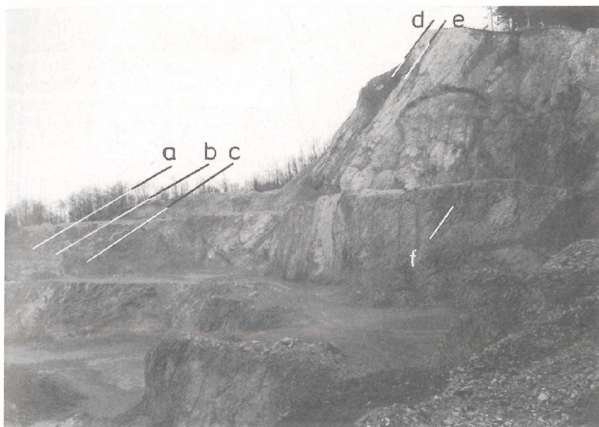
Abb. 8 Steinbruch und Schotterwerk Gogun, Augustdorf-Dörenschlucht. a Flintlage, Grenze zwischen Mittel-Turon (links) und Ober-Turon (rechts), b Inoceramus costellatus / Sternotaxis plana Event, c Tuff T D1 , d Tuff T E , e Mergellage M E , f Hyphantoceras Event.
