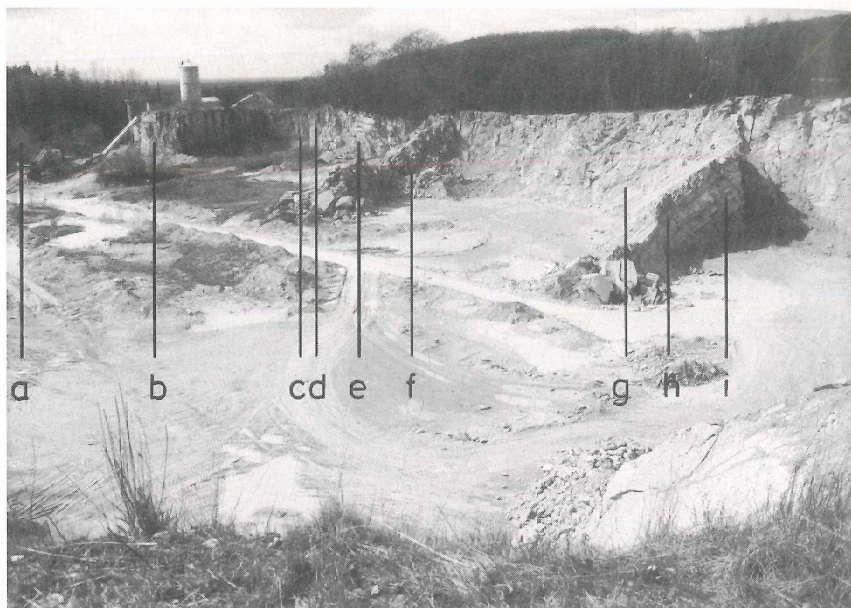
Abb. 5: Steinbruch O. Foerth, Oerlinghausen, West- und Nordseite.
