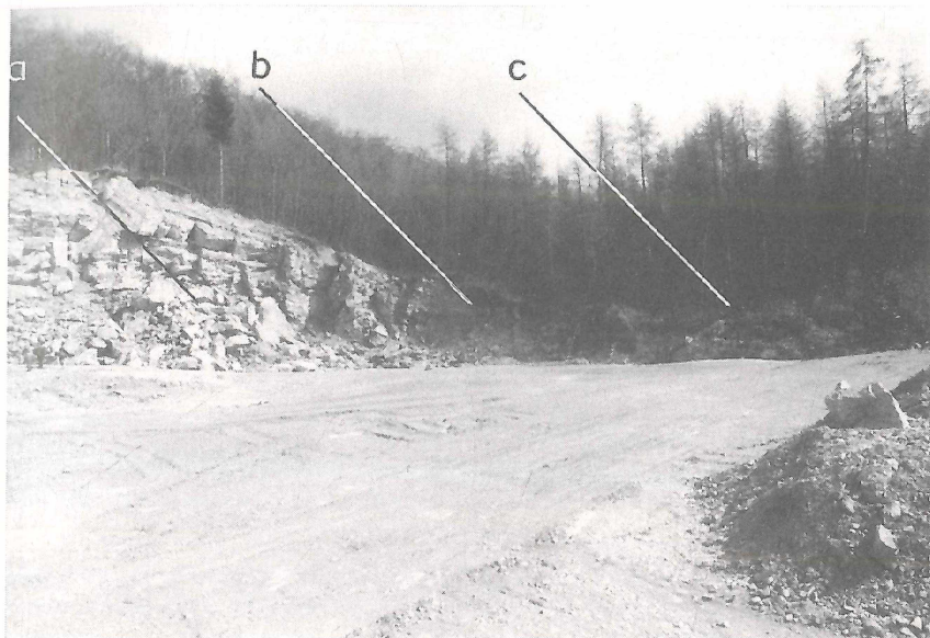
Abb. 4: Steinbruch O. Foerth, Oerlinghausen, nordöstlicher Aufschlußbereich. a Mytiloides Massenvorkommen, b Bereich der Cibolaites sp. & Mytiloides hercynicus Lage, Grenze zwischen der Mytiloides mytiloides Zone (links) und der Mytiloides hercynicus Zone (rechts), c Bereich des Mytiloides hercynicus Events, Grenze zwischen Unter-Turon (links) und Mittel-Turon (rechts).
