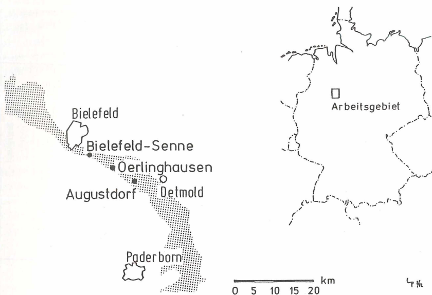
Abb. 1: Lage des Arbeitsgebietes im südöstlichen Teutoburger Wald.
