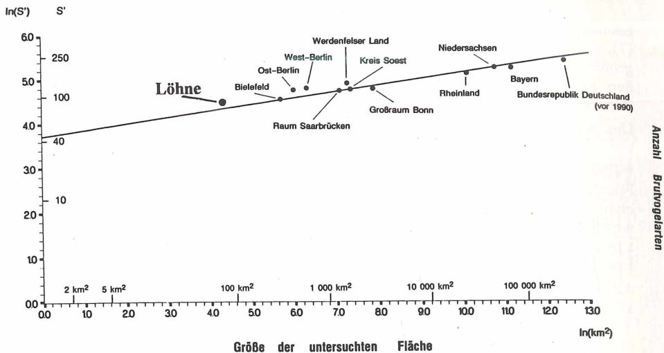
Abb. 3: Die "Art-Areal-Beziehung" für einige ausgewählte Beispiele Nach der Gleichung S' = 41,2 \times A^{0,14} (BANSE & BEZZEL 1984); hier in doppelter logarithmischer Darstellung: \ln(41,2) + \ln(A) \times 0,14 . A = untersuchte Fläche; S' = Anzahl der zu erwartenden Brutvogelarten.
