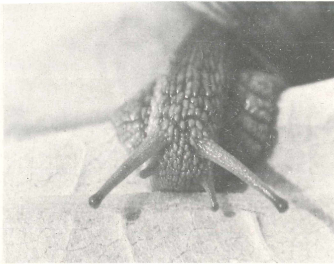
Abb. 1: Normal entwickelte, ausgewachsene Weinbergschnecke Helix pomatia
