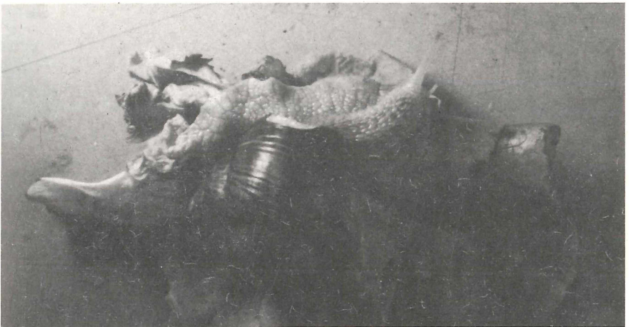
Abb. 2: Helix pomatia mit medianem Augenfühler
