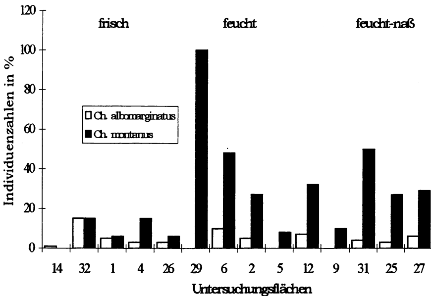
Abb. 3: Verteilung der hygrophilen Arten Chorthippus montanus und Chorthippus albomarginatus an einem Feuchtegradienten
